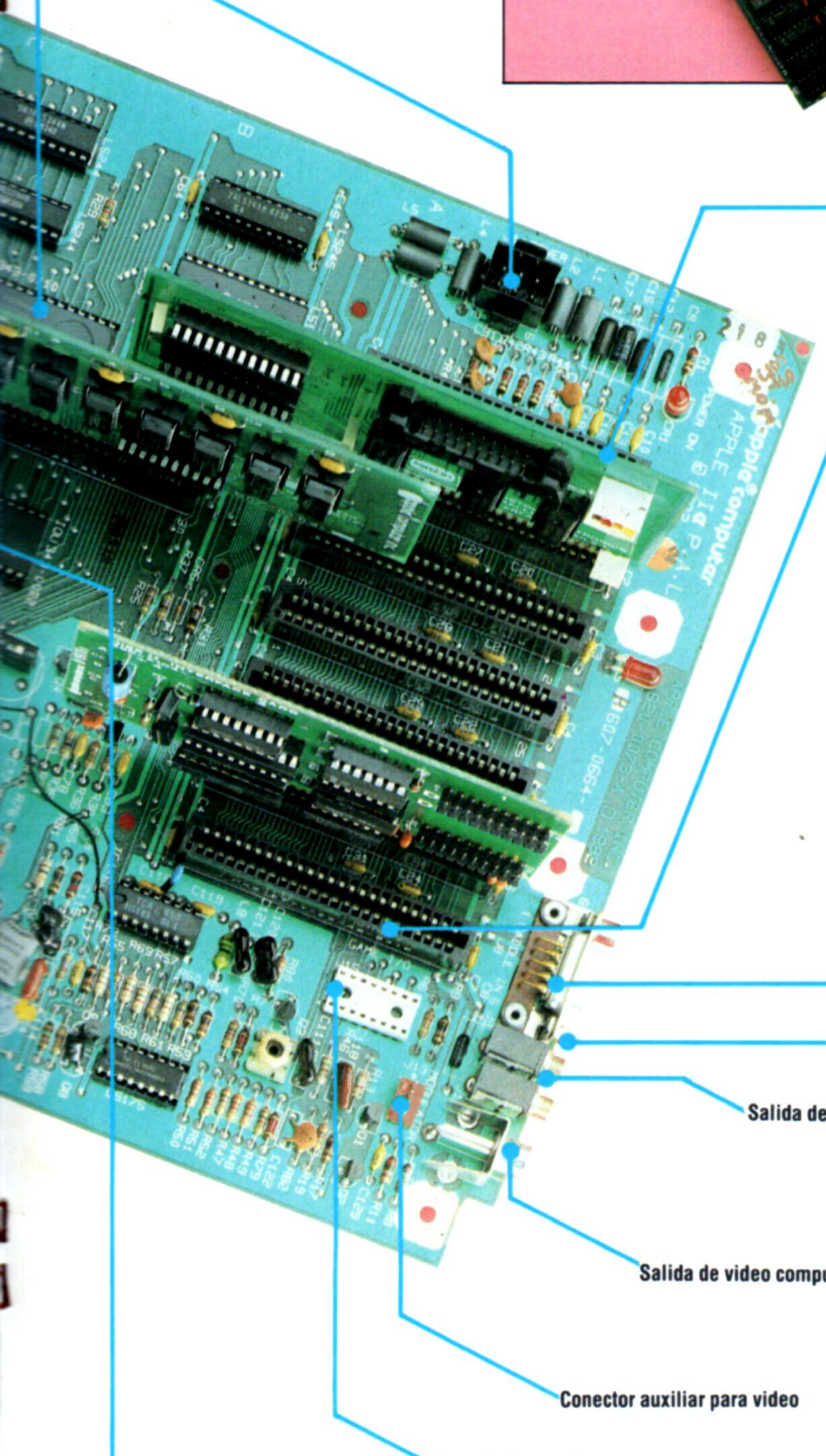
Enchufe-D para juegos El enchufe normal de 16 patillas para conexión de juegos es demasiado frágil para utilizarlo a diario, por lo cual el Apple IIe está equipado con un pequeño enchufe-D en paralelo
