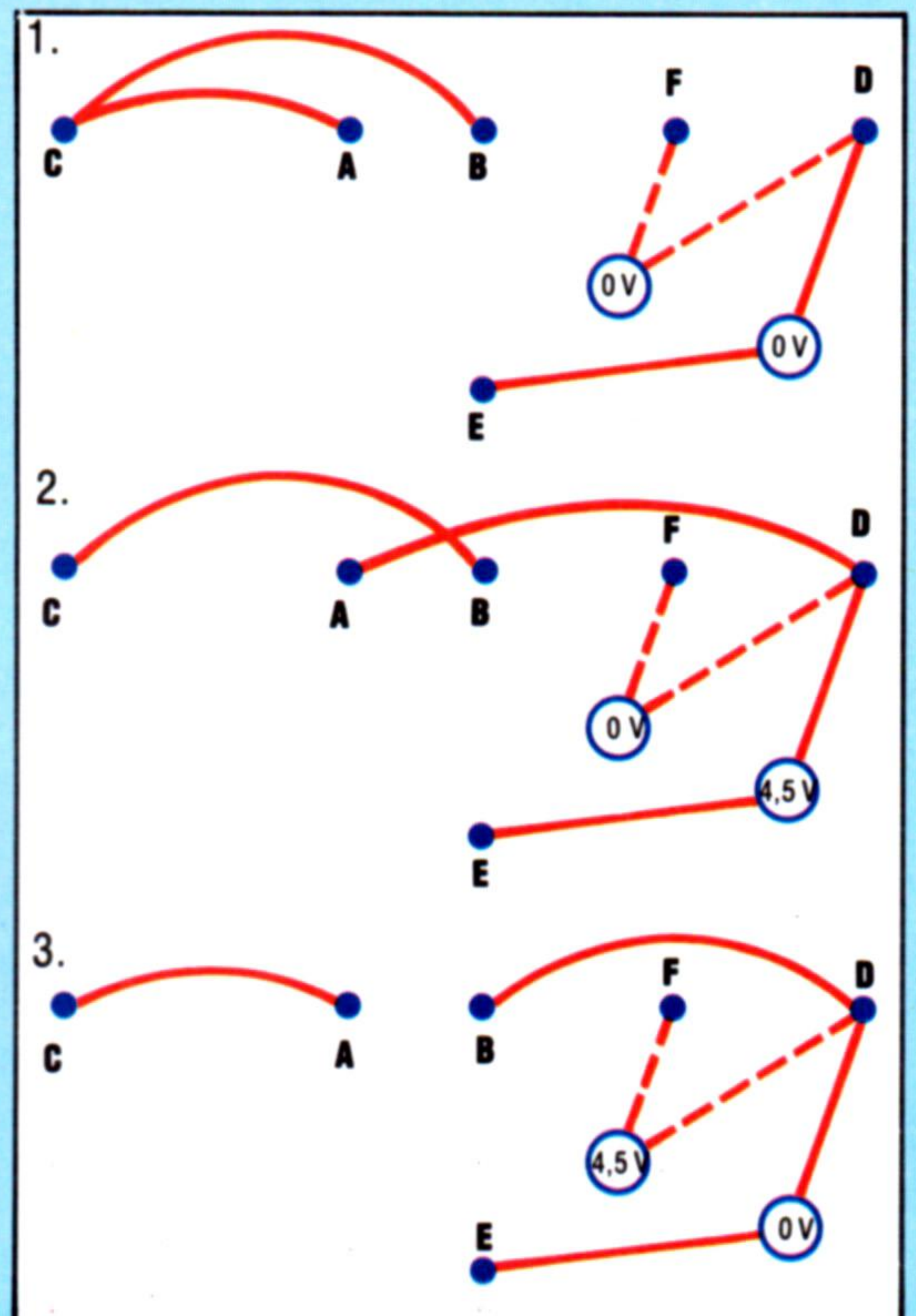
Este diagrama refleja las conexiones de comprobación a efectuar entre los puntos A, B, C y D, y las lecturas correctas que se deben obtener en los puntos E y F en cada una de las tres etapas de prueba
