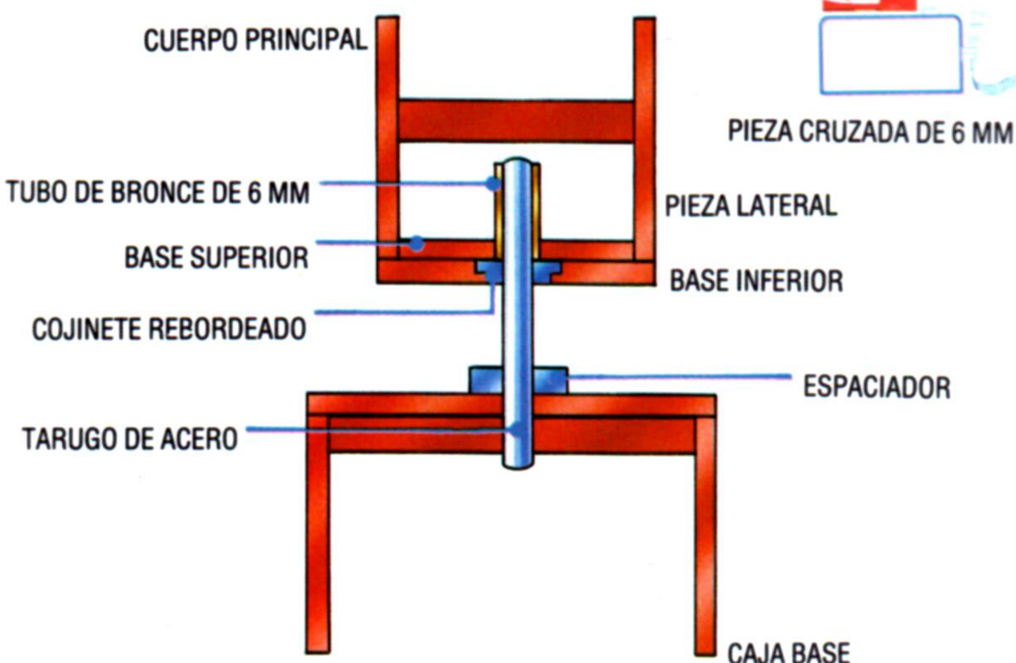
ELEVACION LATERAL
