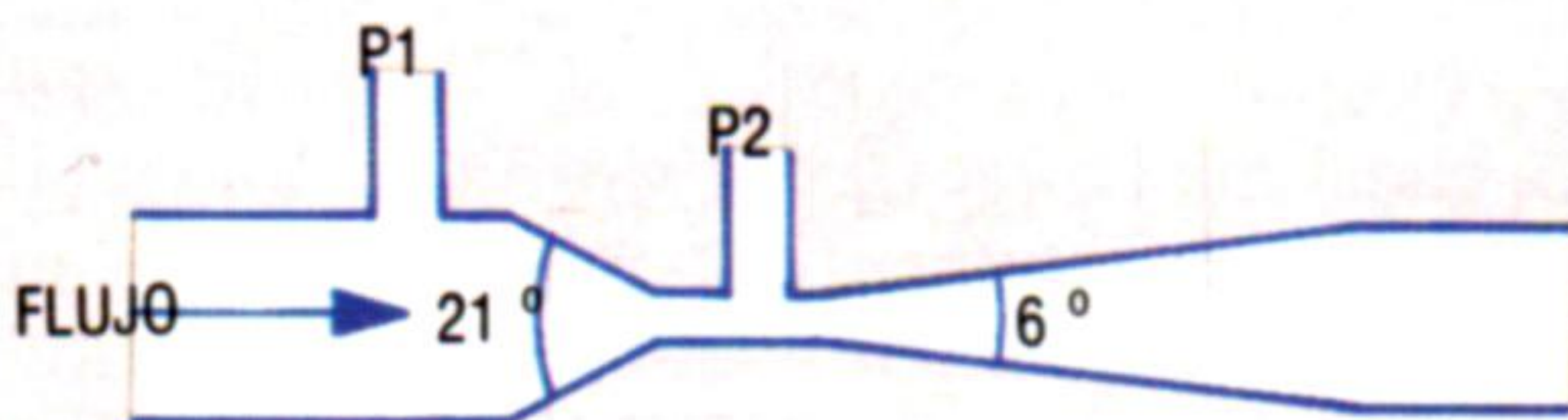
Tubo Venturi
