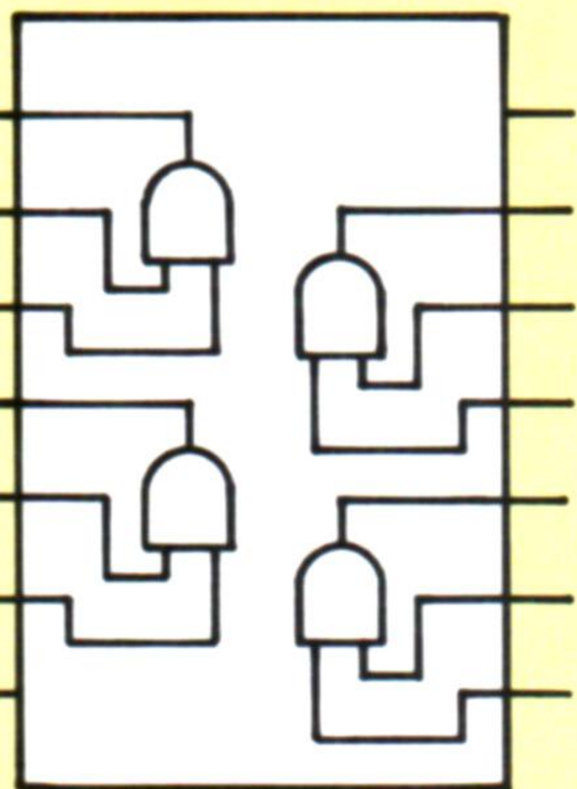
NOR CUAD DE 2 ENTRADAS 74LS02
