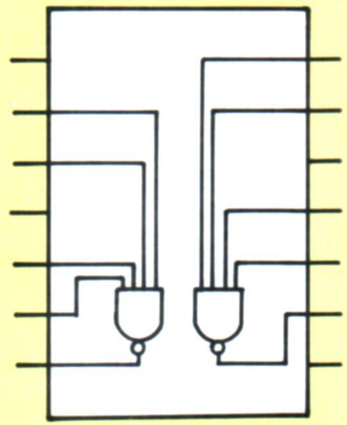
NAND DOBLE DE 4 ENTRADAS 74LS20
