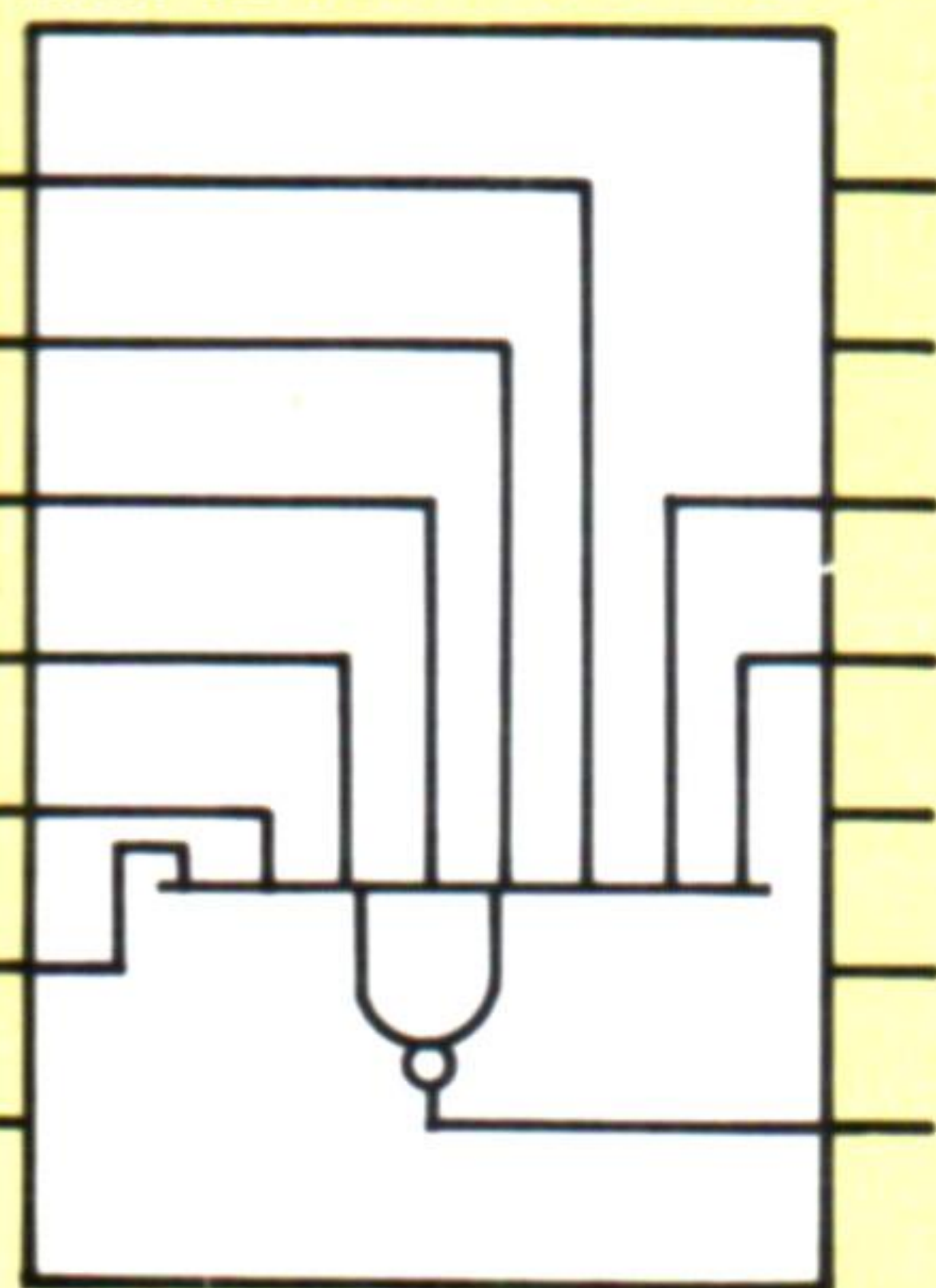
NAND DE 8 ENTRADAS 74LS30
