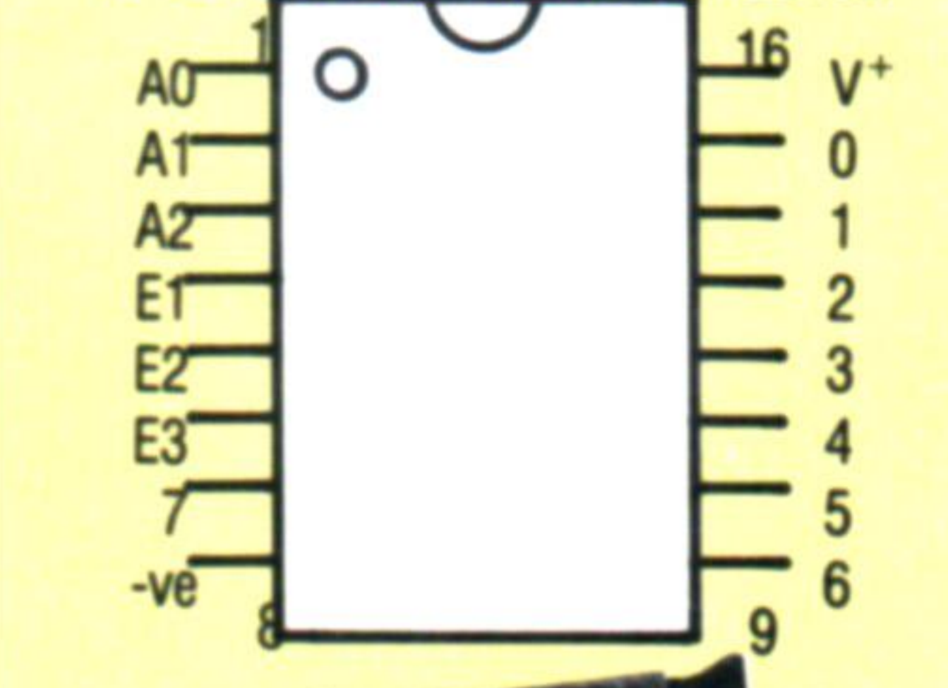
DECODIFICADOR DE 3 A 8 74LS138
