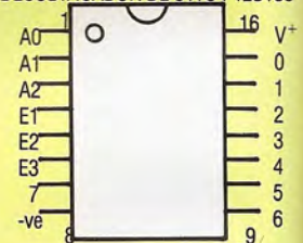
DECODIFICADOR DE 3 A 8 74LS138
