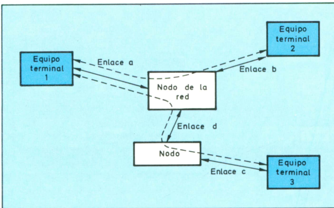
Figura 35. A través del enlace «a» se transmiten simultáneamente dos conexiones lógicas: una entre los terminales 1 y 2, y otra entre el 1 y el 3, gracias al protocolo de red empleado por los tres.
