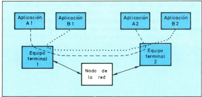
Figura 36. A través de una sola conexión lógica de nivel de red, entre dos terminales 1 y 2 pueden coexistir dos comunicaciones de nivel transporte entre dos aplicaciones distintas.
