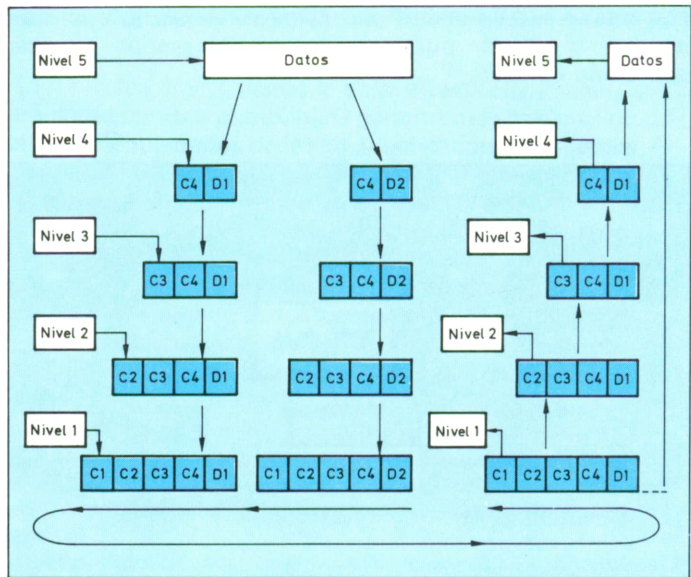
Figura 37. Cada etapa de comunicación añade una cabecera nueva a los datos que recibe del nivel superior, y suprime la cabecera, a ella destinada, de los paquetes servidos por el nivel inferior.
