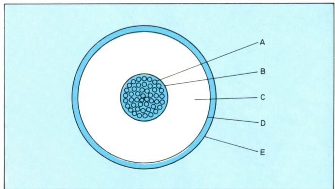
Los cables submarinos requieren una protección adicional que les ayude a soportar la elevada presión a la que están sometidos; A = Hilos de acero; B = Conductor interior; C = Dieléctrico; D = Conductor exterior; E = Cubierta.
