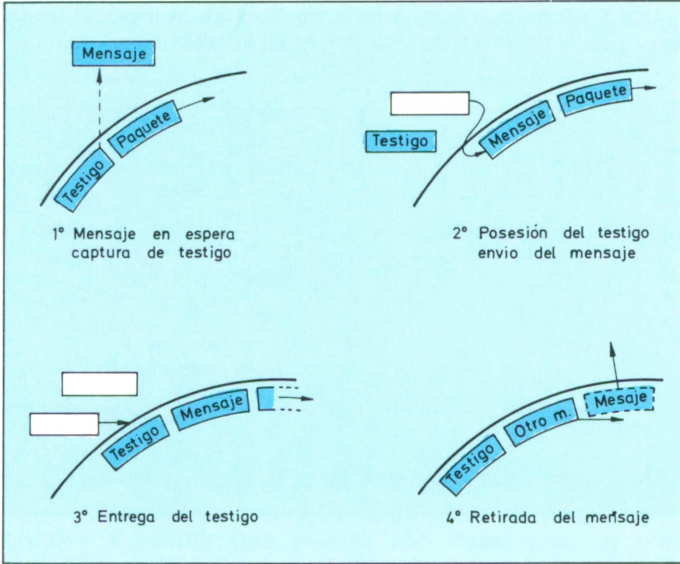
Protocolo de entrega de testigo, en donde se observan las cuatro fases de la impresora.
