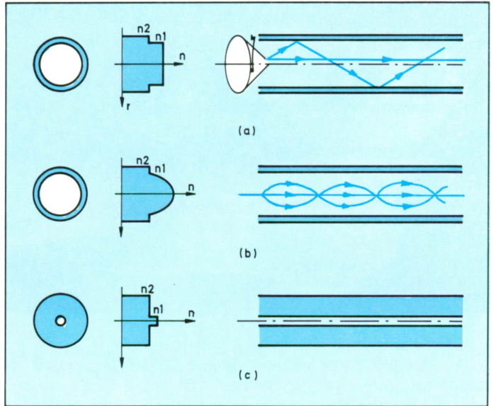
Figura 25. Varios tipos de fibra óptica; a) Fibra óptica multimodo por salto de índice; b) Fibra óptica multimodo por gradiente de índice; c) Fibra óptica monomodo.
