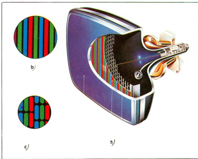
Figura 38. a) Vista interna de un tubo de rayos catódicos tricolor fabricado por la firma Toshiba; b) Detalle de las bandas de luminóforos; c) Disposición de los luminóforos en un tubo de rayos catódicos del tipo autoconvergente.
