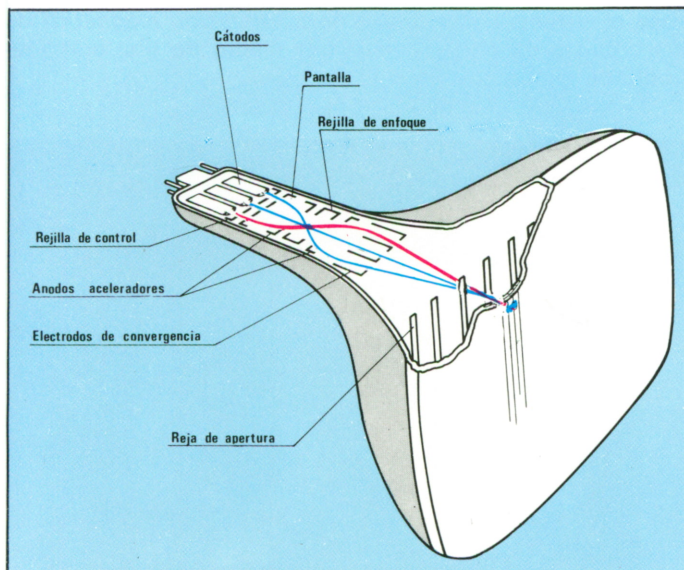
Figura 41. Detalle de la trayectoria seguida por los haces catódicos en un tubo trinitrón. La reja de apertura determina finalmente el lugar del impacto de los haces sobre la pantalla.
