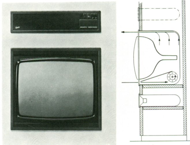
Figura 49. En los televisores que van empotrados en muebles, debe tenerse la precaución de garantizar una buena ventilación del mismo, practicando en el mueble entradas y salidas de aire. En algunos casos, dicha ventilación puede hacerse forzada con un pequeño y silencioso ventilador.
