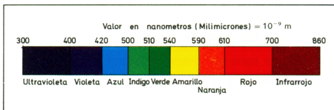
Figura 6. Gama de colores y longitud de onda correspondiente. Así, las diversas tonalidades de rojos, se hallan comprendidas entre 610 y 700 nanómetros.
