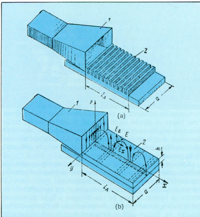
Figura 48. Antena de ondas superficiales.
