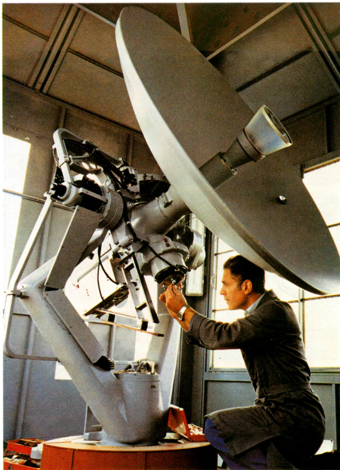
Equipo de enlace de microondas para satélite. Este sistema está provisto de un regulador de desplazamiento de la parábola en cualquier dirección.
