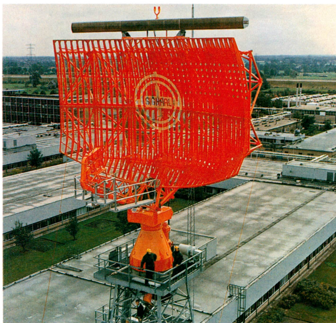
Radar para el aeropuerto de Changi en Singapore, probándose en la factoría de su montaje definitivo.
