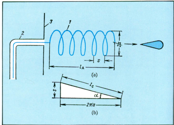
Figura 47. Antena helicoidal representada de forma esquemática, y su diagrama de fuerte directividad.
