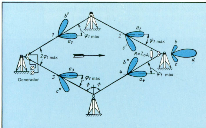
Esquema básico de una antenna rómbica en donde se puede ver la distribución de los lóbulos de radiación.
