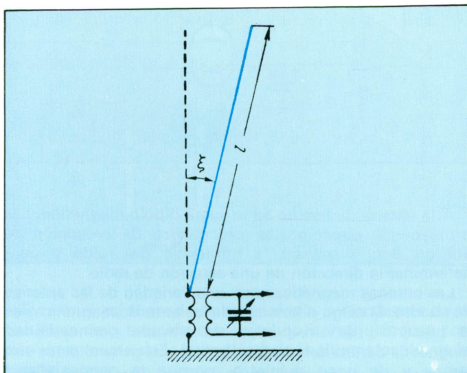
Antena que emplea la posibilidad de un conductor radial inclinado, para modificar con ello la longitud de onda de la misma.
