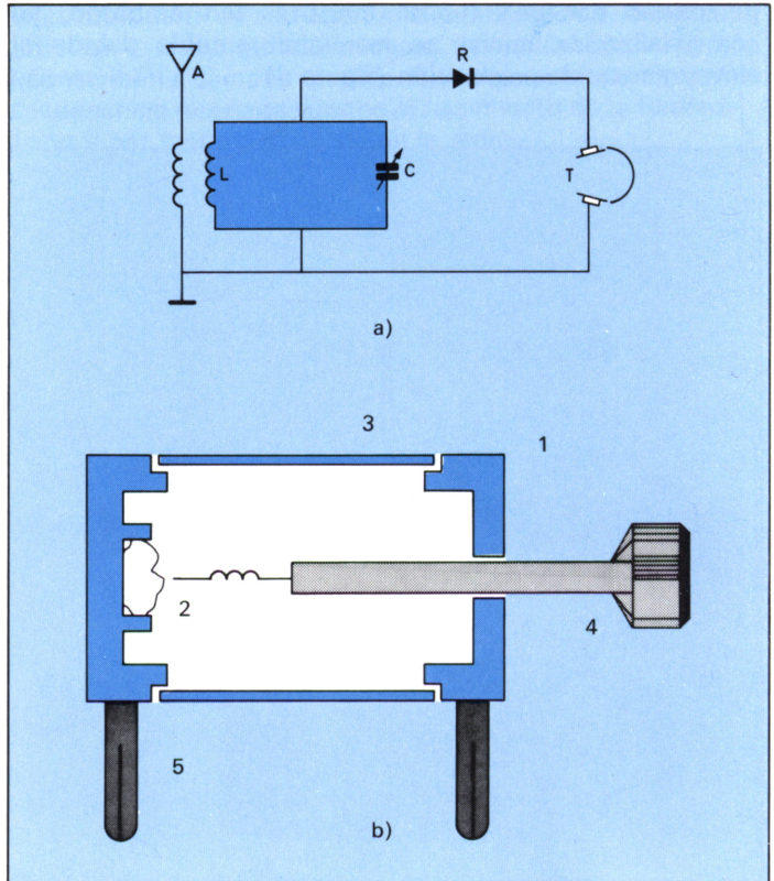
a) Constitución del receptor de galena: A = antena; C = condensador variable; L = inductancia; R = detector de galena; T = auriculares telefónicos; b) Esquema del detector, que consta de: 1 = cápsula metálica; 2 = cristal de galena; 3 = pantalla protectora de vidrio; 4 = mando aislante; 5 = partes de su conexión.
