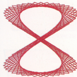
Figures de Lissajous
