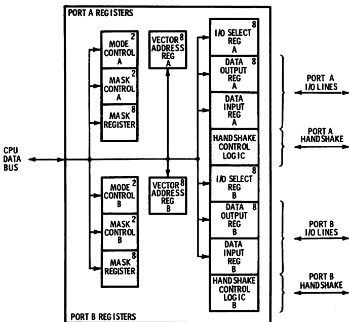
Fig. 8-7. PIO registers.
