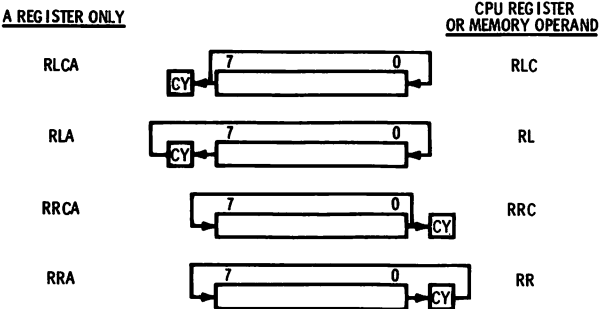
Fig. 12-2. Shift actions.
