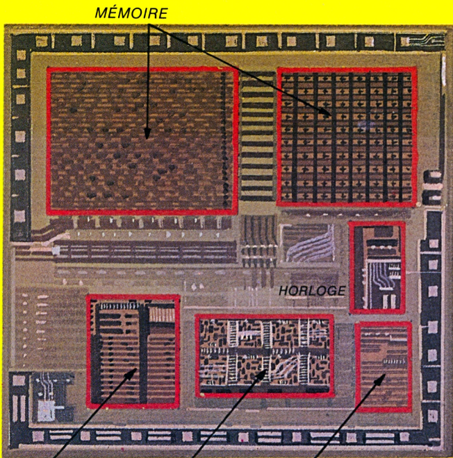
UNITÉ CENTRALE DE TRAITEMENT UNITÉ ARITHMÉTIQUE POINTS D'ENTRÉE ET DE SORTIE DIMENSIONS RÉELLES DE LA PUCE
