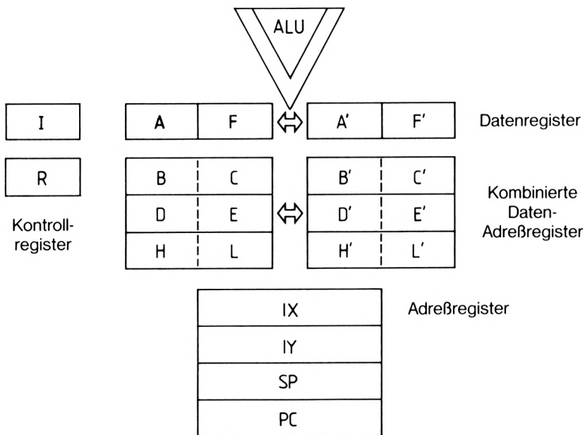
Bild 4.1: Registeraufbau des Z-80-Prozessors
