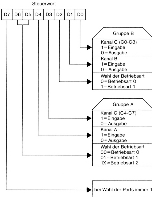
Bild 3.3: Steuerworte und Betriebsarten beim 8255
