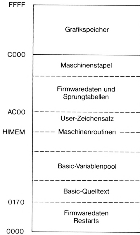
Bild 2.1: Unterteilung des RAM
