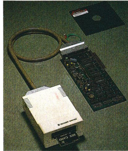
Unidad de lectura-escritura para Software en tarjetas Eprom. La última moda del CeBIT.
