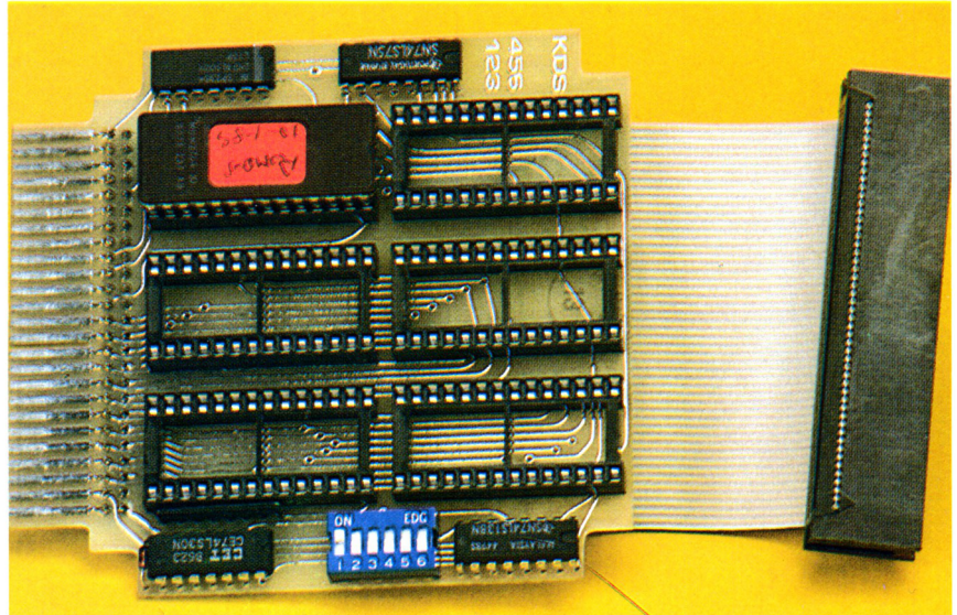
Diferentes conexiones para las ROM's en el interior del interface. En la parte inferior de la placa se pueden observar los switches para seleccionar cada una de las pastillas ROM.
