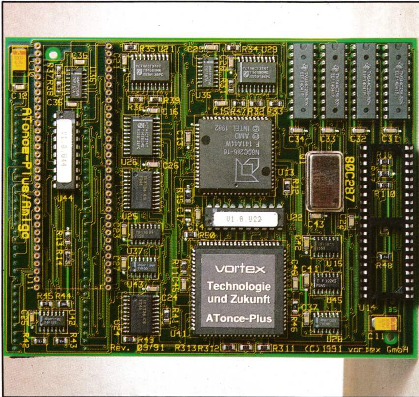
La placa lleva un procesador 286 a 16 Mhz y un zócalo para insertar un coprocesador aritmético.
