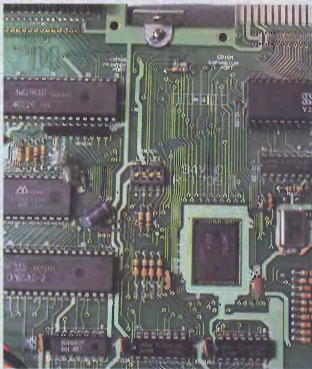
Por el contrario, los modelos recientes de PCW 8256 tienen cuatro microinterruptores (en el centro de la foto), que ejercen la misma función que los puentes anteriores, pero facilitan la tarea de la instalación al no ser necesarias las soldaduras.
