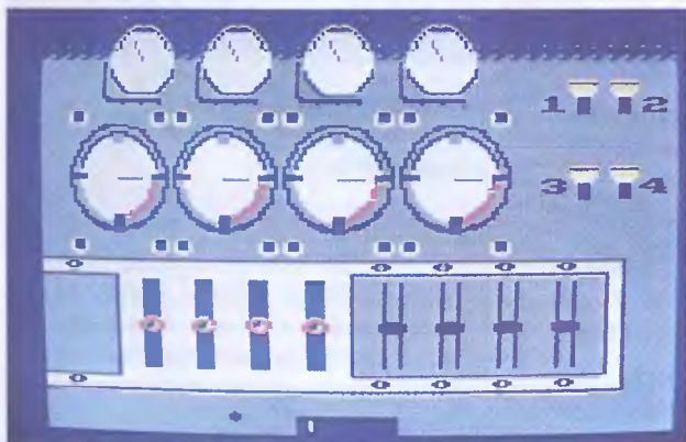
El copiloto controla los cuadros de mandos: en uno están los controles de potencia de los motores y los extintores. En el otro, el control de los flaps y el tren de aterrizaje.
