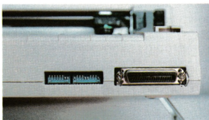
Los microinterruptores, junto al conector Centronics, están accesibles en la partet trasera de la máquina.
