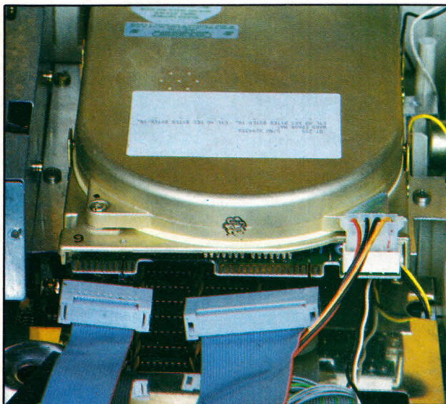
El disco duro se fijará al soporte metálico, con la etiqueta hacia arriba, mediante tornillos. Después realizaremos las conexiones tal y como puede observarse en la fotografía.
