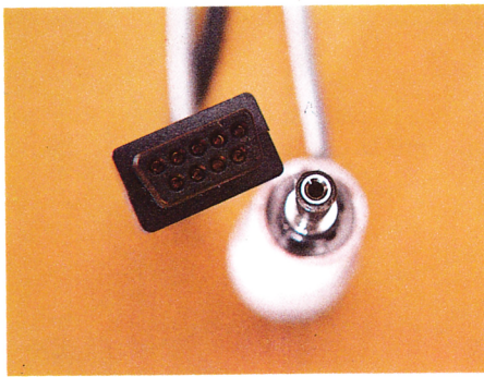
LA CONEXION DE STARMOUSE SE MATERIALIZA A TRAVES DE DOS HEMBRAS: UNA DEL TIPO D, AL PORT DE JOYSTICK, Y OTRA A LA TOMA DE 5V DE LA UNIDAD CENTRAL, A CUYA PARTE TRASERA SE CONECTA A SU VEZ EL CABLE DE ALIMENTACION QUE PARTE DEL MONITOR.
