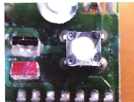
EL MICROINTERRUPTOR QUE SE OBSERVA EN LA FOTO, A LA DERECHA DE UNA DE LAS PAREJAS DE CELULAS, ES EL RESPONSABLE DE LA FALTA DE PRECISION EN EL PULSADOR DEL STARMOUSE; SIN DUDA, SU MAYOR DEFECTO.
