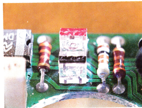
EL INGENUOSO MECANISMO DE CONTROL SE CULMINA CON DOS PAREJAS DE CELULAS FOTOELECTRICAS, QUE DAN FE DEL SENTIDO Y VELOCIDAD DE DESPLAZAMIENTO DEL RATON.
