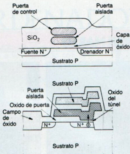
Diferencias de construcción entre celdillas FAMOS y FLTOX en las memorias EPROM y EEPROM, respectivamente.
