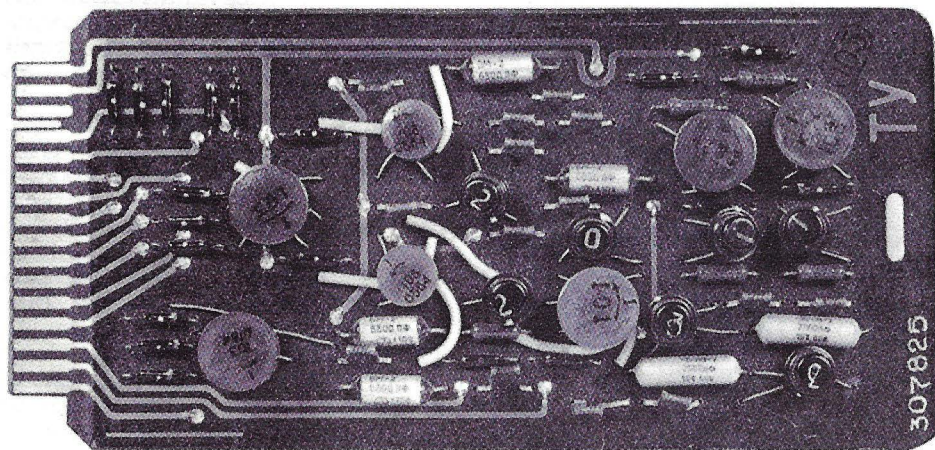
Tarjeta del Minsk-2, uno de los ordenadores de propósito general más utilizados en la URSS durante los años sesenta.
