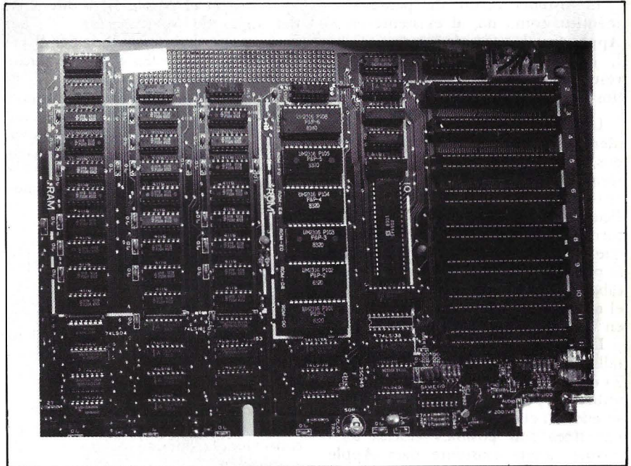
La similitud de esta tarjeta central con la observada en el microordenador Apple II+ es grande realmente. Dispone también de los 8 slots destinados al alojamiento de las numerosas tarjetas de ampliación del sistema actualmente comercializadas por gran número de fabricantes.
