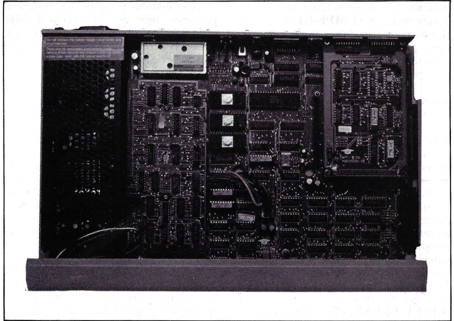
La tarjeta principal del MPF-III tiene una configuración sustancialmente distinta a la observada en el Apple II . La caja metálica de la parte superior es el modulador de video para utilizar un televisor corriente. Las tarjetas destinadas a los periféricos se sitúan paralelamente a la tarjeta principal, como se ve en la foto.
