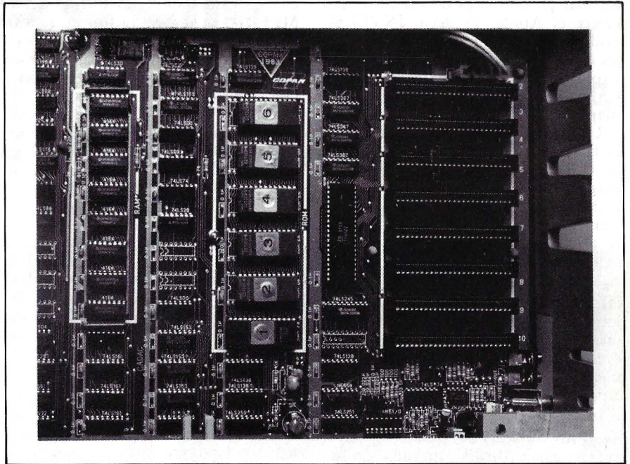
En la parte posterior de la tarjeta principal de circuito impreso del Base 64/A se pueden observar los 8 slots para las tarjetas de expansión del sistema. Se puede observar que algunos de los circuitos integrados van soldados directamente a la placa, en lugar de estar insertados en zócalos.
