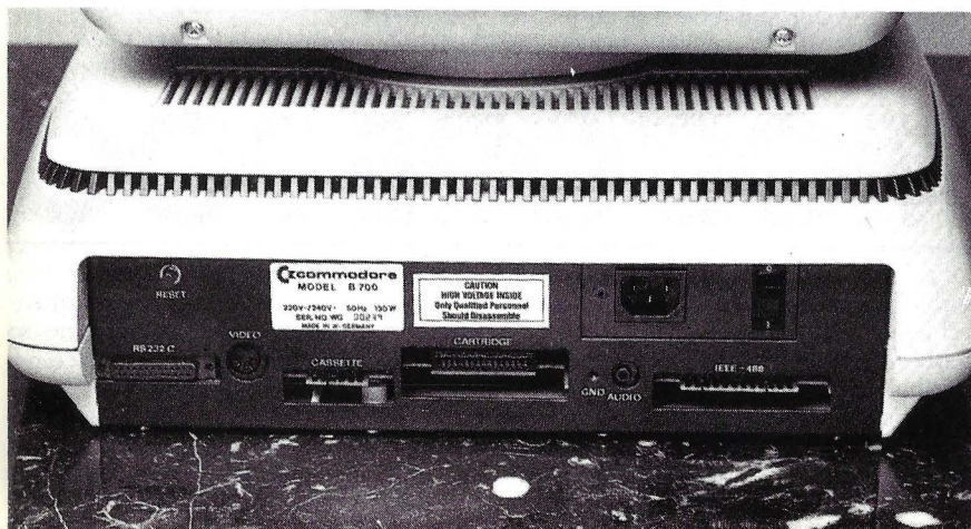
La parte posterior del Commodore 700.
