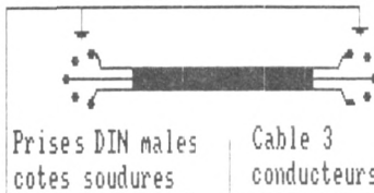
fig.4 Cable de liaison CPC MINITEL
