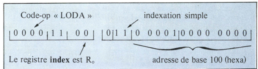
Fig. 2. - Découpe des instructions à trois octets, permettant l'adressage indexé.
