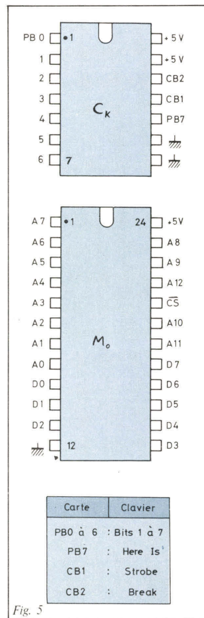
Fig. 5. - Liaisons à effectuer entre le connecteur M 0 (Basic), le connecteur CK (clavier) et la carte micro-ordinateur.
