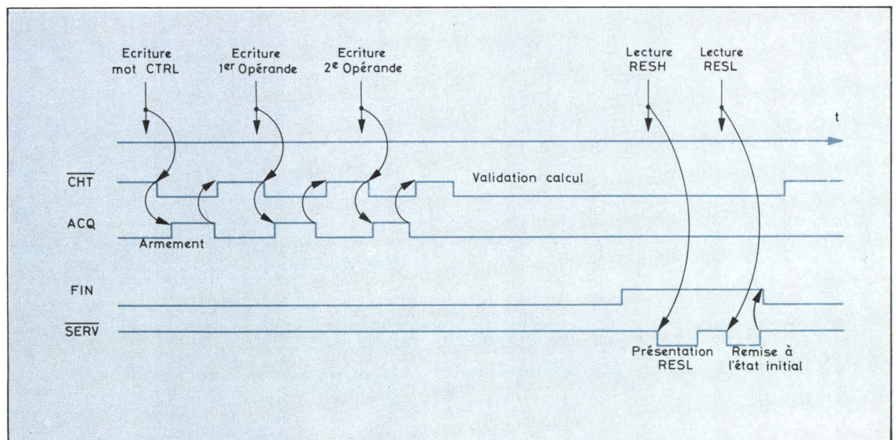
Fig. 2. - Chronogramme général représentant le fonctionnement de MULDIV.
