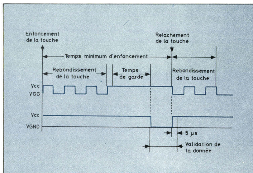
Fig. 3. - Diagramme du temps entre l'enfoncement et le relâchement d'une touche; lors de l'enfoncement d'une touche, les contacts mis en présence peuvent rebondir; un temps de garde est alors nécessaire avant la validation de la donnée.
