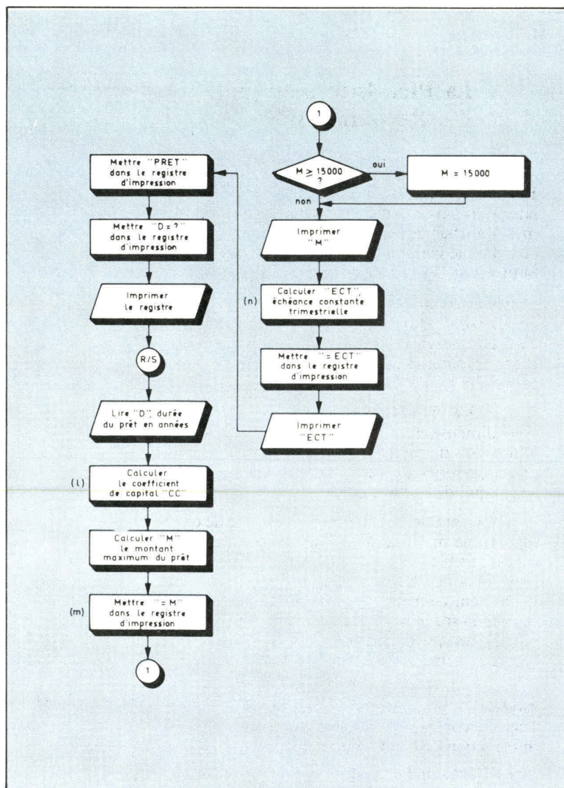
Fig. 2. - Organigramme de la phase « crédit » du PEL.
