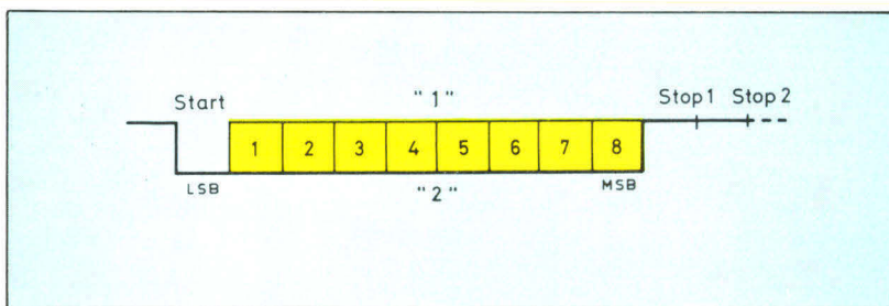
Fig. 1. - Format d'enregistrement du standard « Kansas City ».
