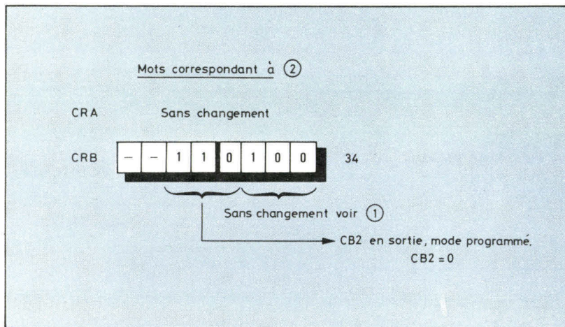
Fig. 7. - Un nouveau mot de commande CRB est écrit définissant ainsi CB2 comme une sortie en mode programmé.
