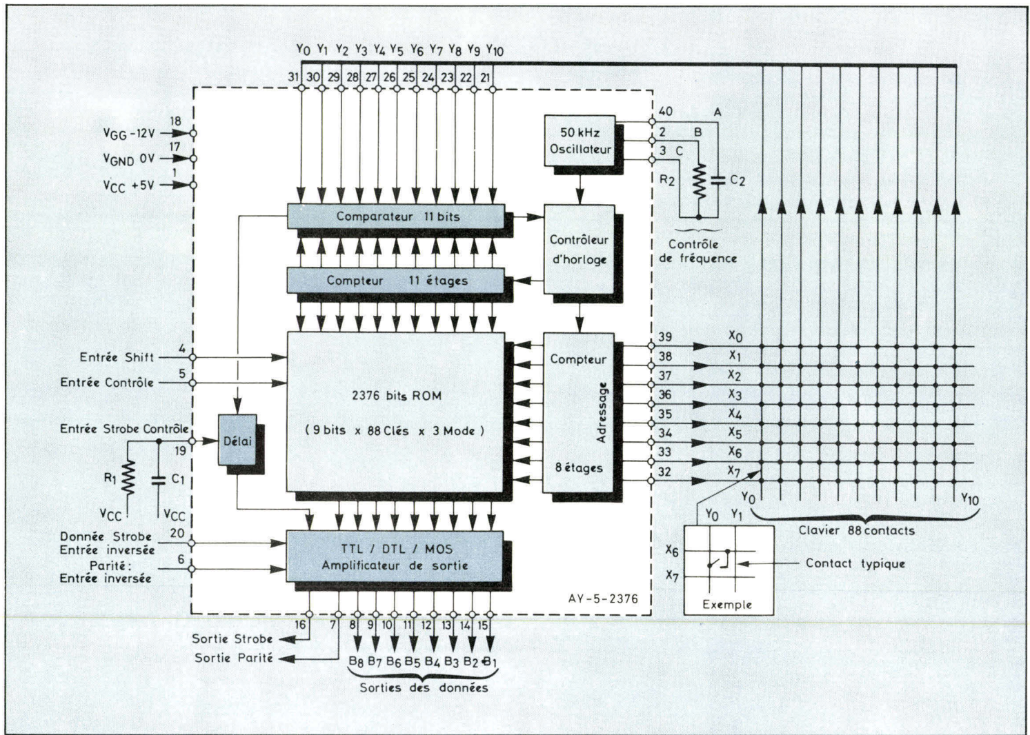
Fig. 1. - Schéma synoptique du circuit encodeur de clavier AY-5-2376 de General Instrument.
