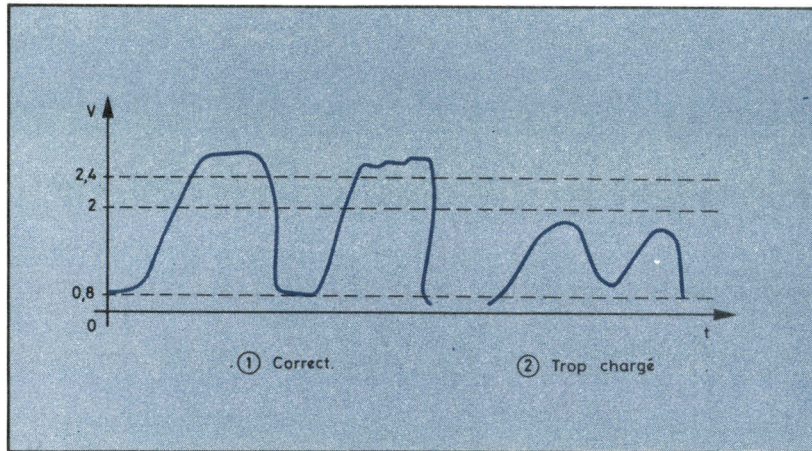
Fig. 1. - Un exemple de cause de mauvais fonctionnement hardware. Lorsque l'on veut commander plus de 10 entrées TTL avec une seule sortie TTL (2), la tension ne descend pas assez bas dans l'état 0 (elle reste > 0,8 V) et ne monte pas assez haut dans l'état 1.
