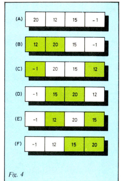
Fig. 4. - Les différentes étapes du classement depuis la ligne A (combinaison initiale) jusqu'à la ligne F (combinaison finale). Les parties en couleur sont les cases perméutées. Les lignes sans changement ne sont pas représentées.
