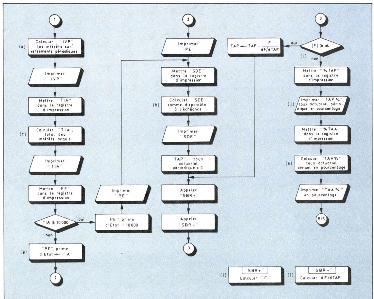
Fig. 1 (suite et fin). - Calcul des intérêts sur versements périodiques, de la somme disponible en fin d'Épargne et du Taux Acturiel Annuel.
