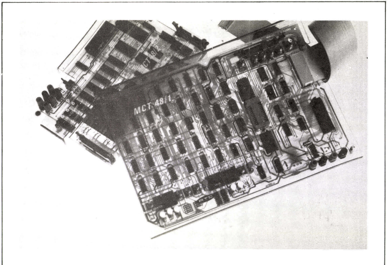
Photo 2. - Ensemble de test et de mise au point pour micro-ordinateurs 8048-MCT 48 (Document RTC).
