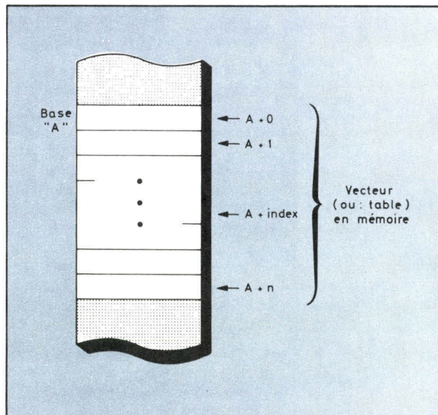
Fig. 1. - Dans une table (ou vecteur), chaque position mémoire est repérée par son numéro relatif, ou index, par rapport à une adresse choisie : la base.
