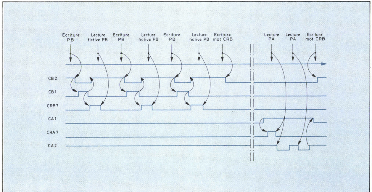
Fig. 4. - Diagramme des temps relatif au PIA.
