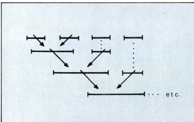
Fig. 2. — Ce tri de fichier par interclassement utilise des fichiers partiels triés au fur et à mesure qu'ils se présentent.
