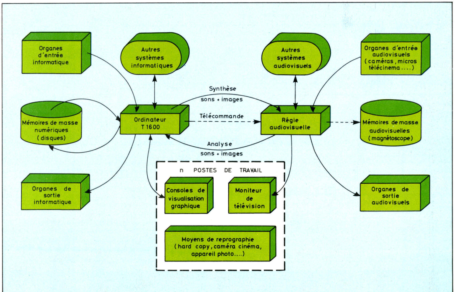
Fig. 1. - Architecture du Système Multimedia Conversationnel SMC permettant de marier les techniques informatiques et audiovisuelles. Le sous-ensemble informatique, centré sur l'ordinateur T 1600, est représenté sur la partie gauche. Le sous-ensemble audiovisuel centré sur une régie de télévision analogique figure à droite du dessin.
