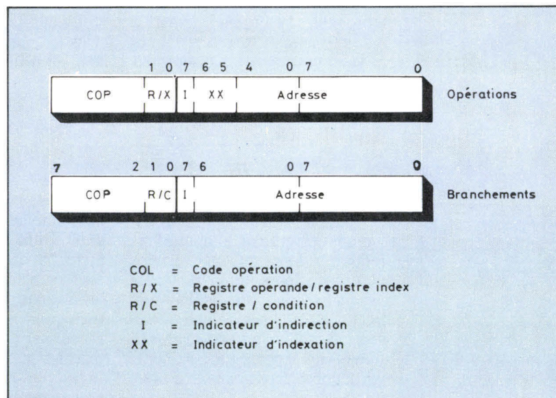
Fig. 2. - Découpe des instructions à trois octets, permettant l'adressage indexé.
