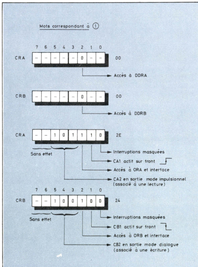
Fig. 6. - Programmation des registres CRA et CRB , correspondant à la phase d'initialisation.
