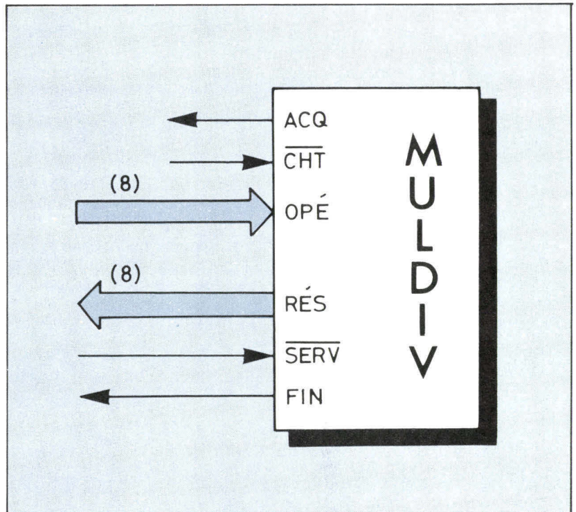
Fig. 1. - Dans notre exemple, le périphérique utilisé est un multiplieur-diviseur 8 bits par 8 bits rapide car microprogrammé.
