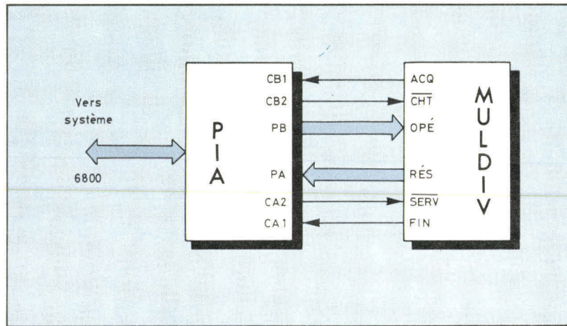
Fig. 3. - Schéma de branchement de MULDIV à un PIA.
