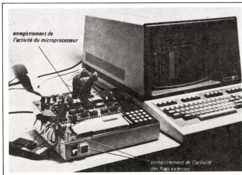
Photo 6. - Tests et analyse en temps réel à l'aide d'un système universel d'aide au développement Tektronix.
