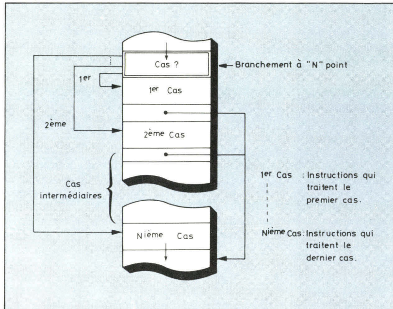
Fig. 3. - Structure : « Dans le cas... ». Dans le premier cas, il faut faire ceci ; dans le deuxième, faire cela ; dans le troisième... etc., etc.
