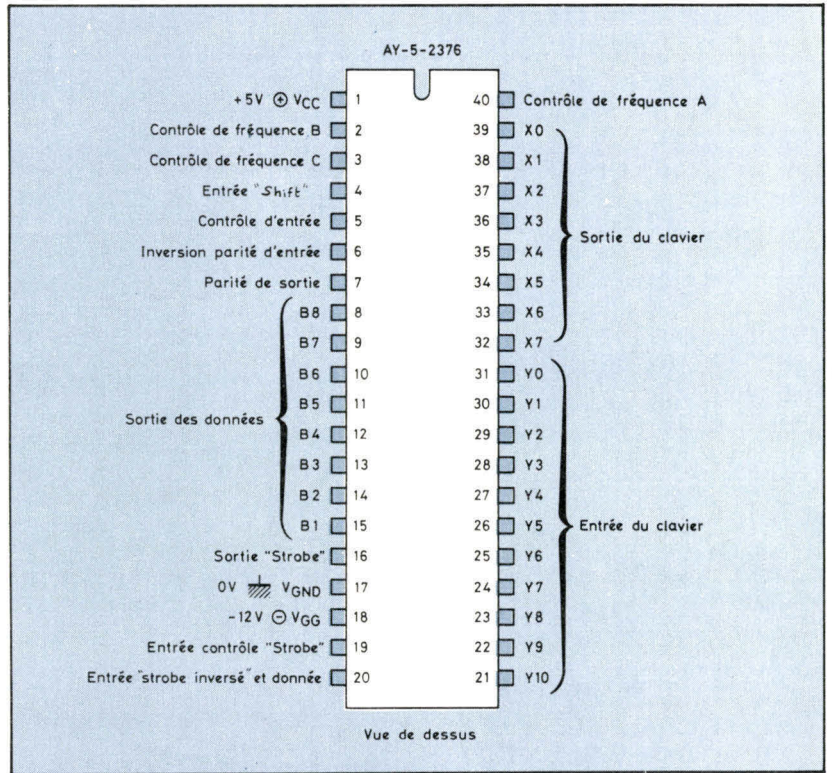
Fig. 2. - Brochage du circuit intégré AY-5-2376.
