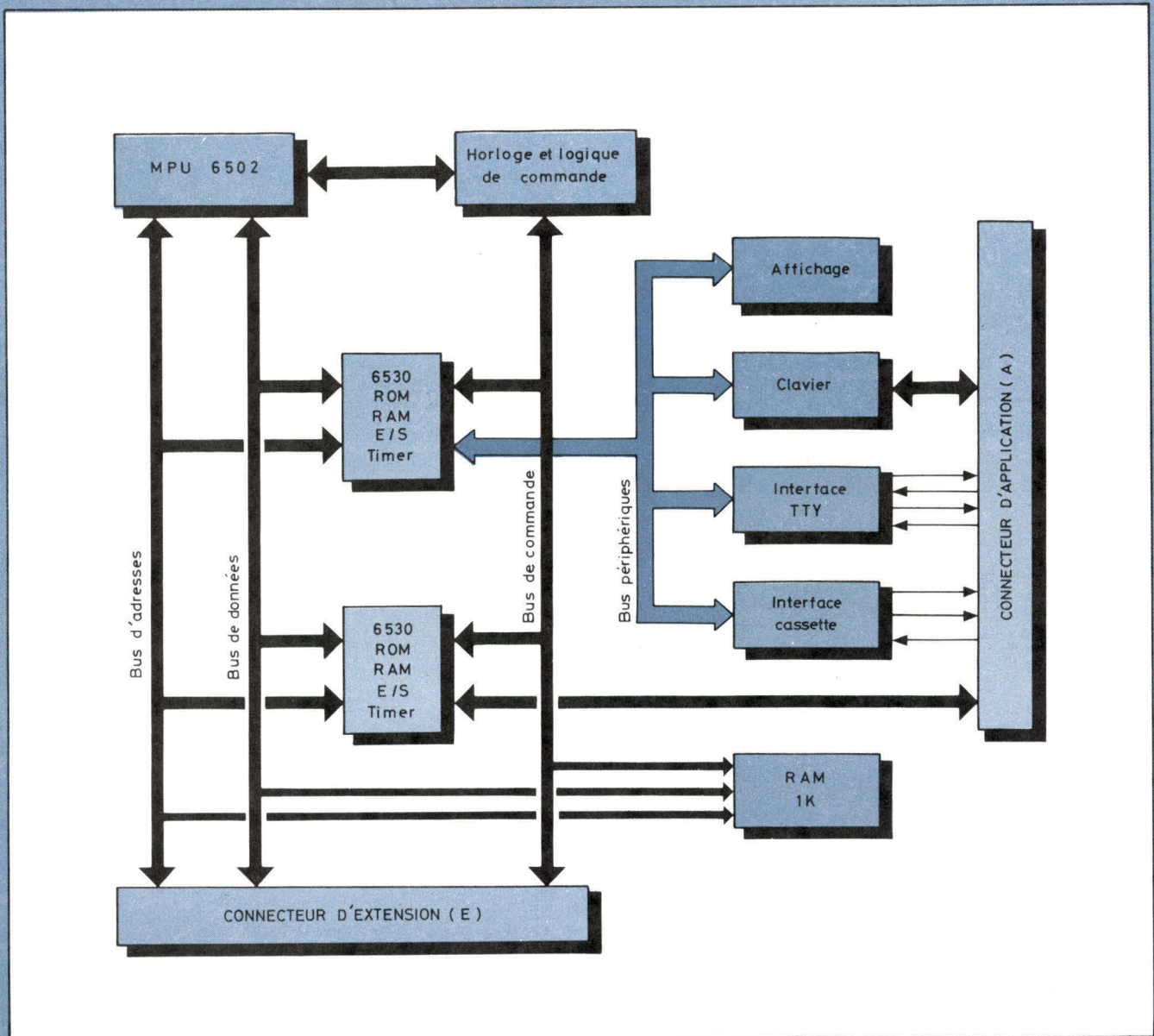
Fig. 1. - Schéma synoptique du KIM.
