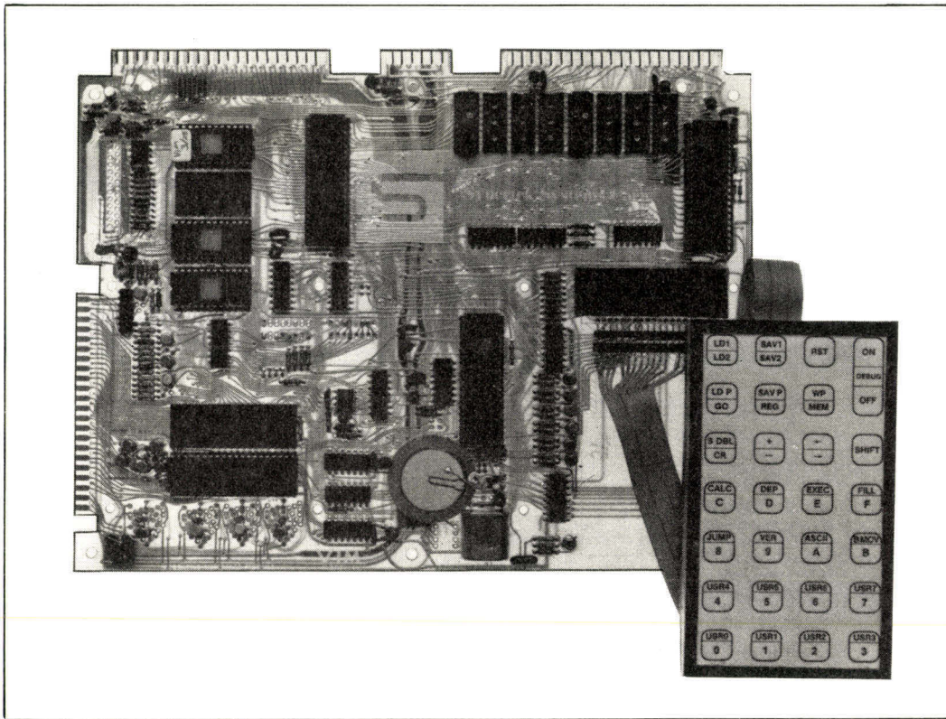
Photo 1. - Le VIM 1 : micro-ordinateur sur une carte construit par la société Synertek.
