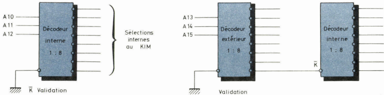
Figure 2 : Décodage des adresses :
