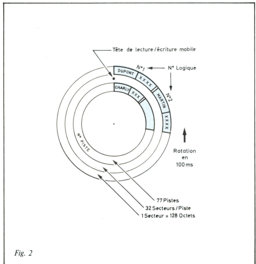
Fig. 2. - En positionnant directement la tête de lecture/écriture sur la piste où se trouve l'enregistrement cherché, on accède directement à celui-ci. C'est l'organisation directe.
