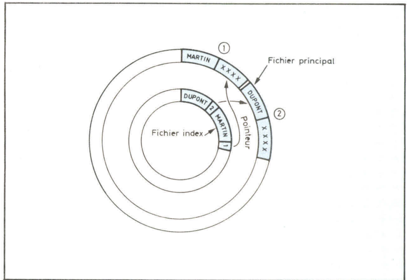
Fig. 5. - L'index de taille réduite, donc exploré rapidement, peut être lui-même enregistré sur disque.
