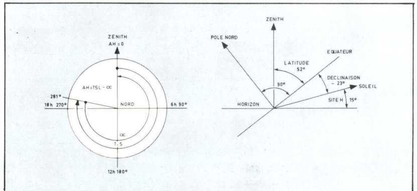
Fig. 4. - Passage solaire au méridien de Greenwich. Représentation des principales grandeurs pour les données suivantes : Latitude : 52^\circ Nord, longitude : 0^\circ , date : 1 er janvier 1980, heure : 12 h 03, TSL = 281^\circ . Ascension droite = 281^\circ . Angle horaire = 0^\circ . Déclinaison = -23^\circ . Site = 15^\circ . Azimut = 180^\circ . On constate une différence entre l'angle horaire exprimé en degrés décimaux et sa valeur en heures, minutes et secondes : cette différence de 180^\circ vient du fait que la référence 0^\circ est prise sur le méridien, à 12 heures locales.
