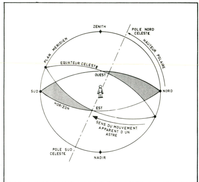
Fig. 1 B. - Pour pouvoir repérer les directions de l'espace, un observateur utilise une sphère de rayon arbitraire : la sphère céleste dont il occupe le centre.
