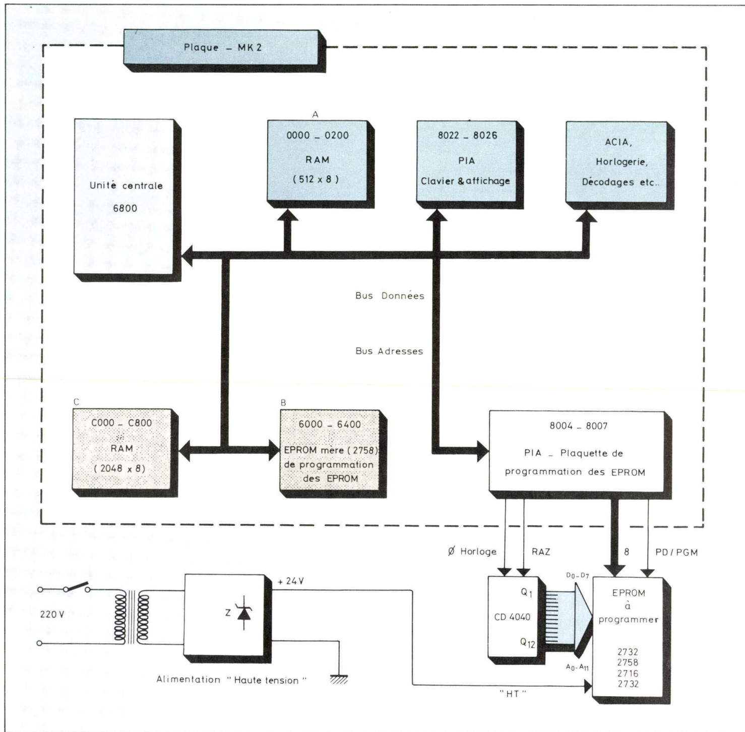
Fig. 2 b. - Synoptique général de l'ensemble : kit d'initiation MK 2 avec son coupleur d'entrée-sortie PIA, système de programmation des EPROM et alimentation « haute tension ».
