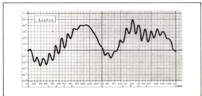
Fig. 3. - Courbe d'erreur 1978-1979 : Cette courbe d'erreur a été établie pour l'heure de passage du soleil au méridien de Greenwich, le 1 er et le 15 de chaque mois. Date de référence : 1 er janvier 1978. Documents d'origine : connaissance des temps 1978 et 1979. L'erreur maximum ne dépasse pas + 50 secondes d'arc et reste inférieure à la limite indiquée : + / - 1 minute d'arc.
