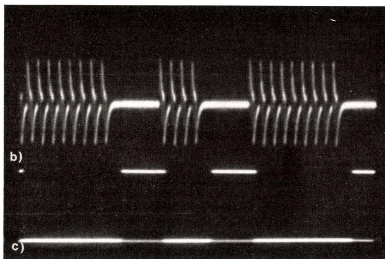
Photo 1. - a) Signal observé à l'oscilloscope au point « A » (fig. 1) du ZX 81 « émetteur ». Neuf impulsions transmettent un « 1 » tandis que quatre un « 0 ». b) Signal prélevé au point « B » (fig. 1) du ZX 81 « récepteur ». c) « Echo vidéo » présent au point A du ZX 81 « récepteur ». Durant un train d'impulsions, le signal vidéo est à « 0 » (= noir); entre deux trains d'impulsions, celui-ci est à « 1 » (= blanc). Ce signal est à l'origine des rayures que vous pouvez observer à l'écran lors du chargement d'une cassette.
