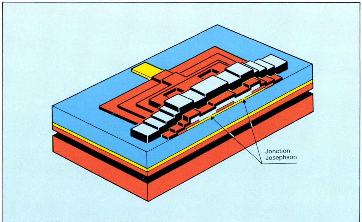
Fig. 17. - La structure schématique d'un dispositif à deux jonctions Josephson donne une idée de l'empilement des couches des circuits logiques et des mémoires.
