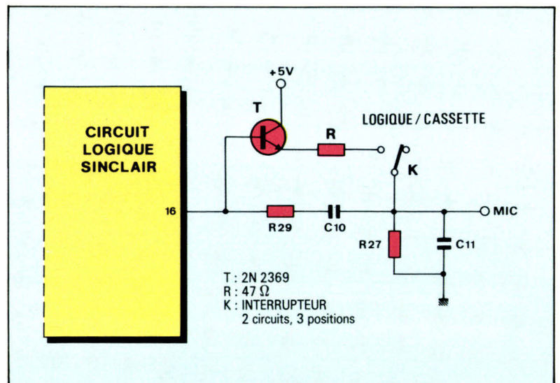
Fig. 3. - L'interrupteur assure l'émission de données vers le magnétophone à cassette ou vers la mémoire vive du second ZX 81.
