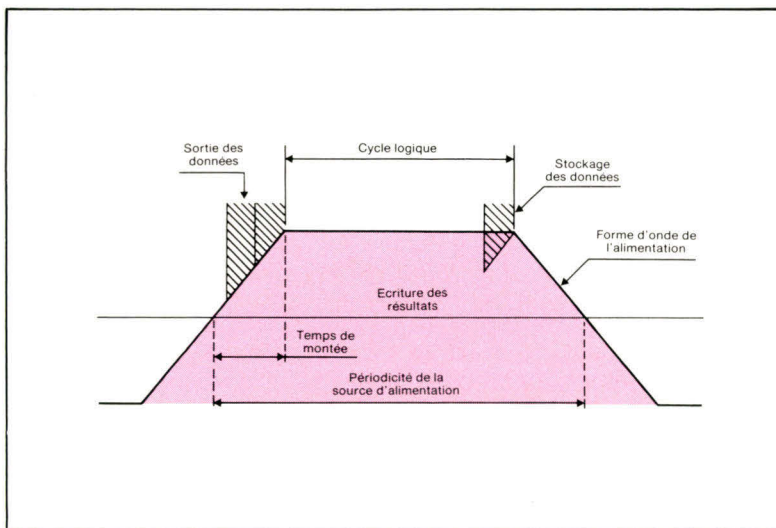
Fig. 15. - Forme d'onde de l'alimentation des circuits Josephson. Une source sinusoidale sert en même temps d'alimentation et d'horloge pour la synchronisation.
