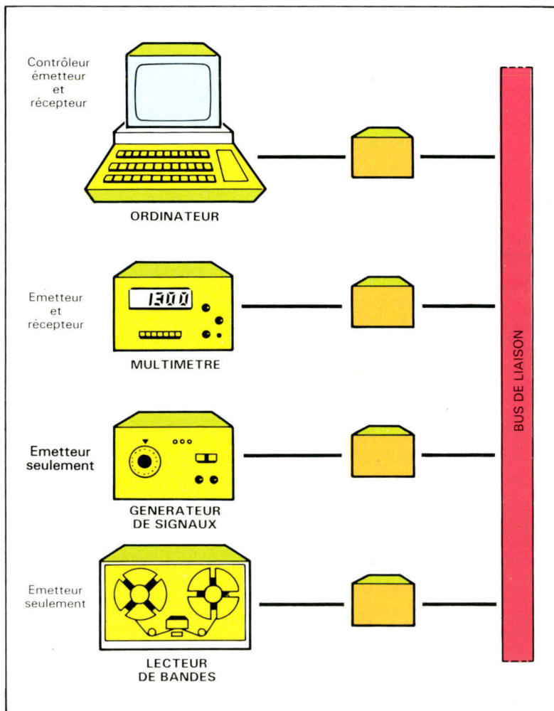
Fig. 2. - Comportement (récepteurs ou émetteurs) des périphériques d'une chaîne de mesures automatiques.
