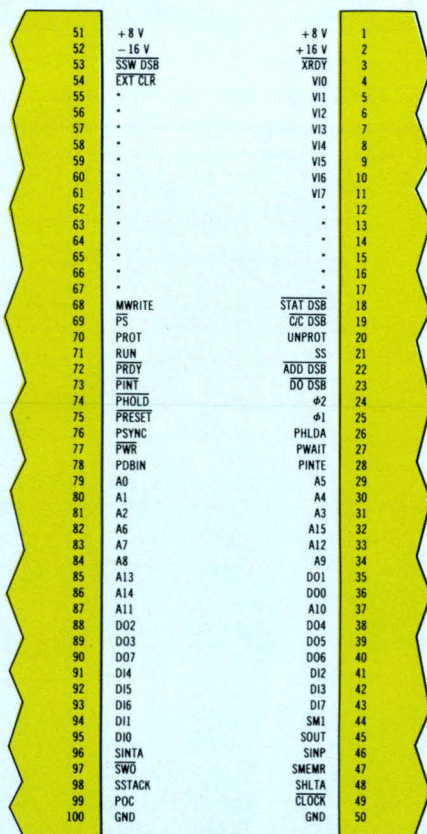
Fig. 13. - Les signaux du bus S100.
