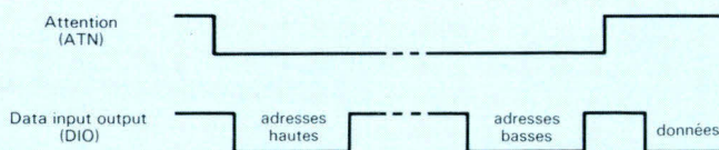
Fig. 3. - Chronogramme illustrant le multiplexage « adresses-données » du bus IEEE 488.
