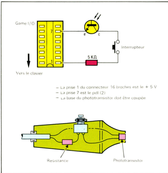
Fig. 2. - Schéma électrique et montage du « Light-Pen ».
