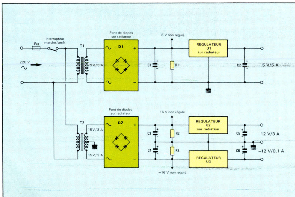
Fig. A. - Schéma de l'alimentation de Vegas.
