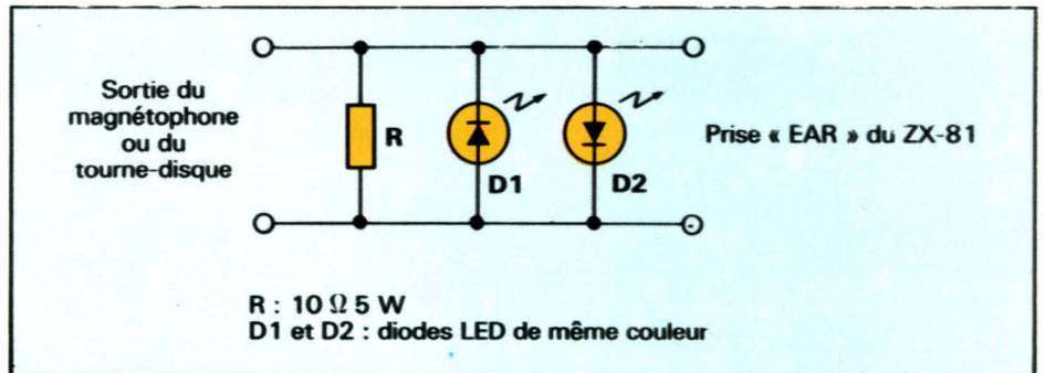
Fig 2 - Deux diodes LED montées « tête bêche » signalent, par leur seuil d'éclairement, que le volume est correct.
