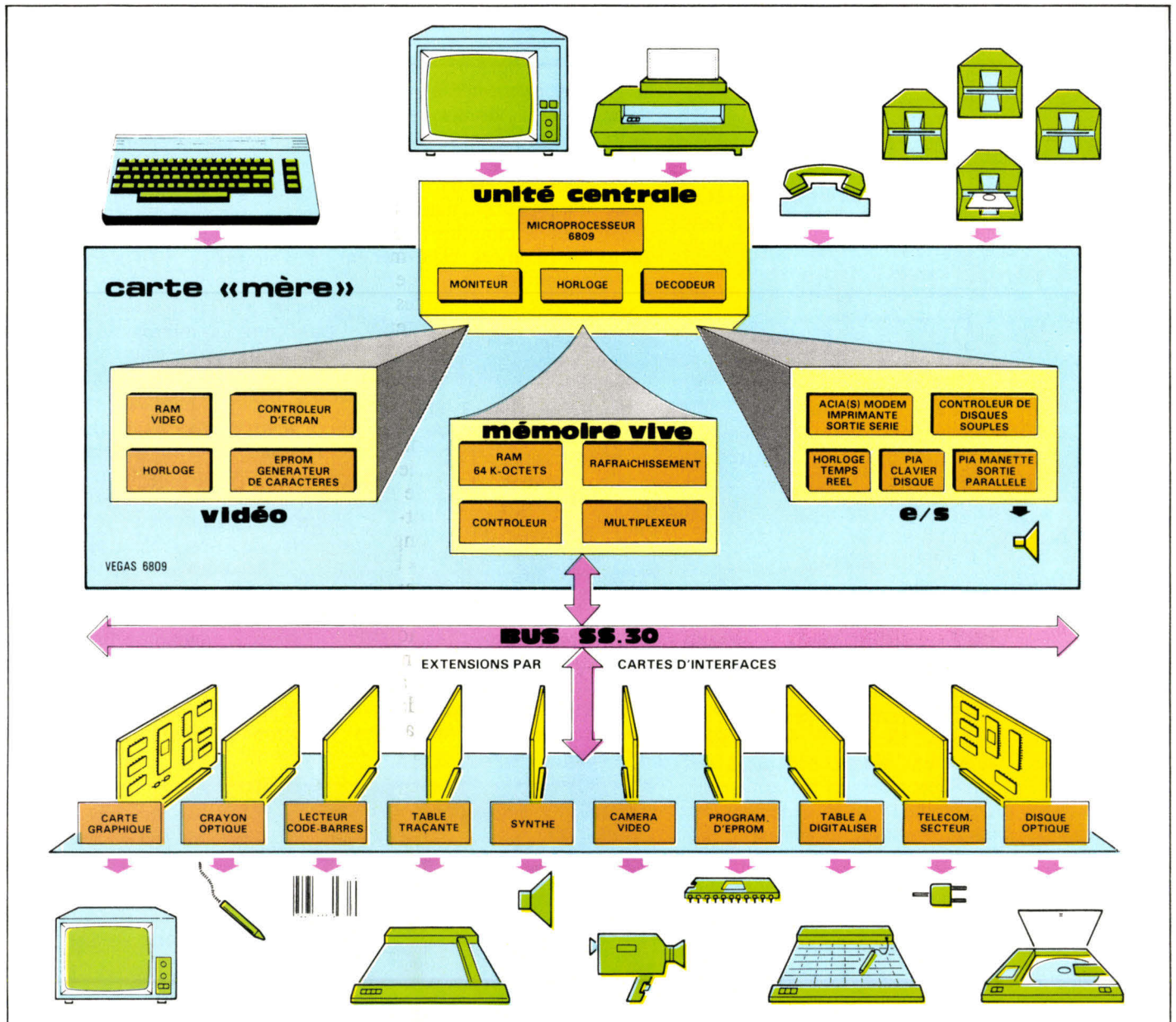
Fig. 1. - Le synoptique de Vegas 6809. Le système avec les extensions possibles. Les quatre parties principales (unité centrale, vidéo, mémoire vive et entrées-sorties) ont été réparties sur la carte « mère ». Au-dessus de celle-ci, il est possible de placer une carte-support au format du bus SS 30, permettant ainsi de connecter au micro-ordinateur dans le même boîtier jusqu'à huit cartes d'interfaces diverses. Huit autres cartes peuvent aussi y être reliées, qui seront, quant à elles, disposées dans un coffret annexe.
