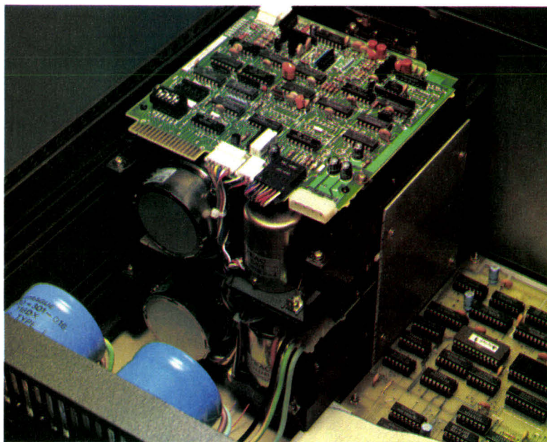
Deux lecteurs de disquettes 5 1/4" prennent place aisément dans le boîtier.
