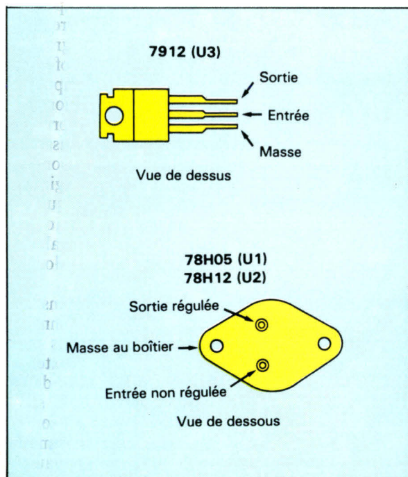
Fig. B. - Brochage des boîtiers des régulateurs.
