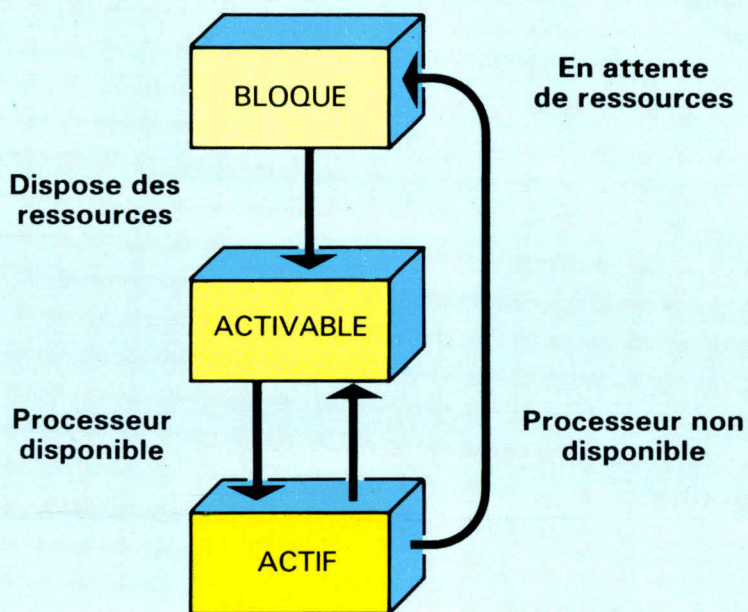
Fig. 3. - Les trois états d'un processus : actif, activable et bloqué. Ces états s'enchaînent suivant la disponibilité ou l'absence de ressources ou de processeurs adéquats.
