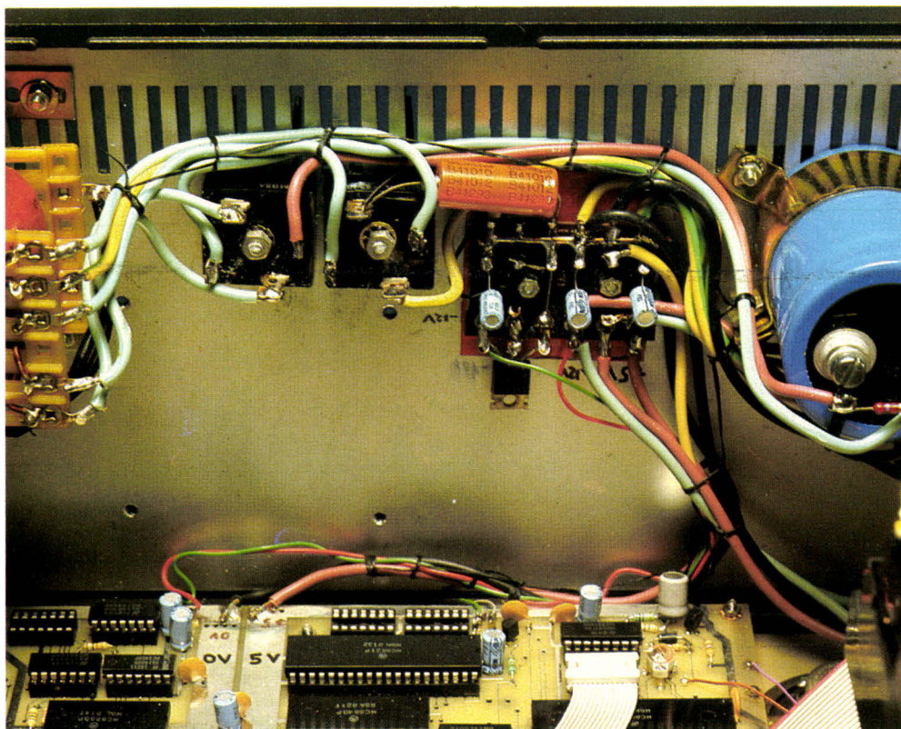
Une simple plaque de douze cosses convient pour réaliser les connexions de l'alimentation.
