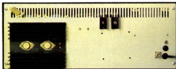
Les radiateurs en « U » assurent le refroidissement des ponts de diodes, le troisième, de taille plus importante, supporte les régulateurs U 1 et U 2 .
