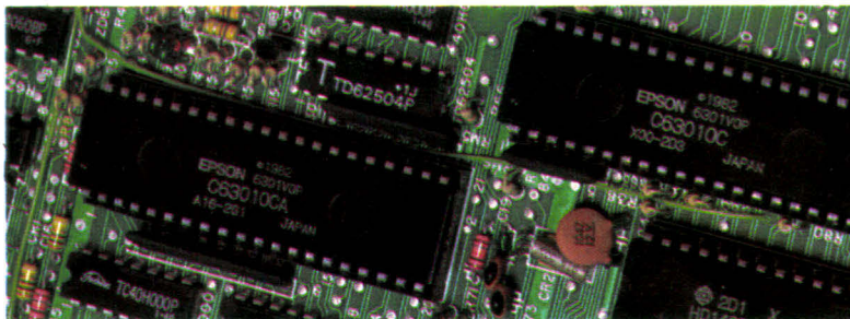
Le HX-20 possède deux microprocesseurs 6301, dont l'un est « l'esclave » de l'autre.
