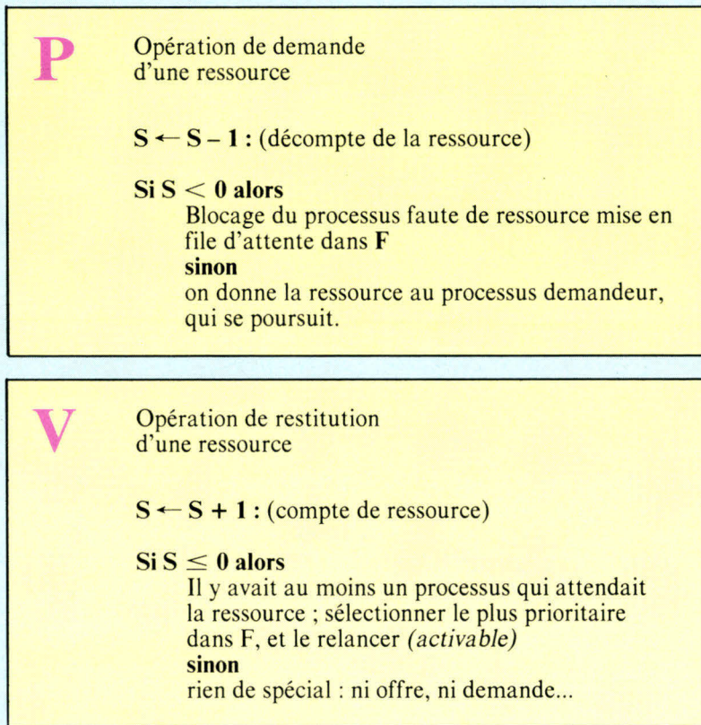
Fig. 4. - Les deux sémaphores P et V. Utilisés de manière courante dans tous les systèmes d'exploitation modernes, ils servent à gérer la répartition des ressources suivant la demande des processus.
