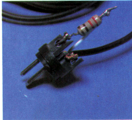
Au cas où vous choisiriez d'utiliser la prise « haut-parleur » de votre tourne-disque, il vous faudra insérer une résistance de protection afin de ne pas endommager l'étage de sortie de l'amplificateur de votre tourne-disque.
