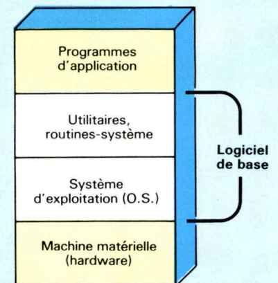
Fig. 1. - Le modèle en couche d'un système d'exploitation correspond à une hiérarchie de fonctions : le niveau le plus bas est celui de la machine réelle, le plus haut celui des programmes d'application.
