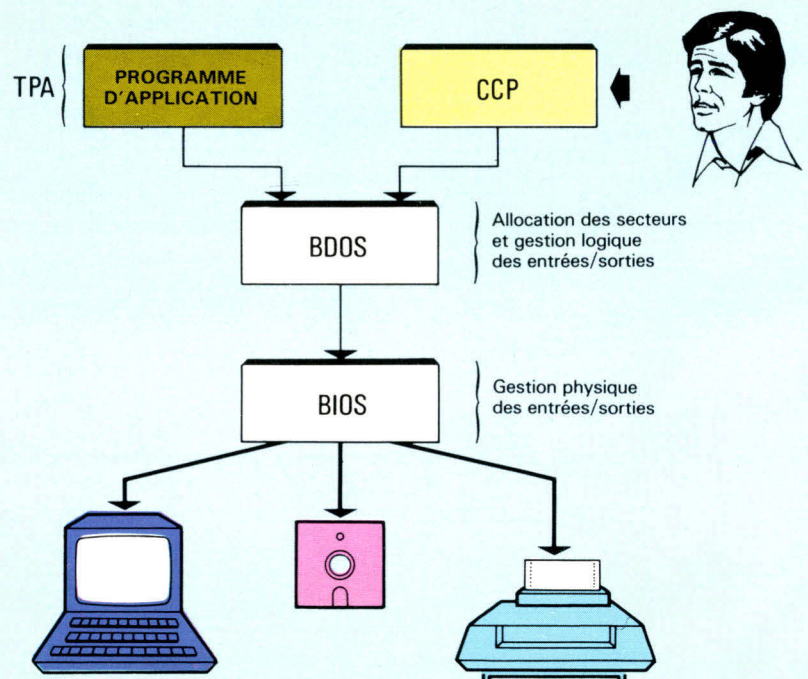
Fig. 2. – CP/M est fonctionnellement constitué de trois modules : le CCP, le BDOS et le BIOS.
