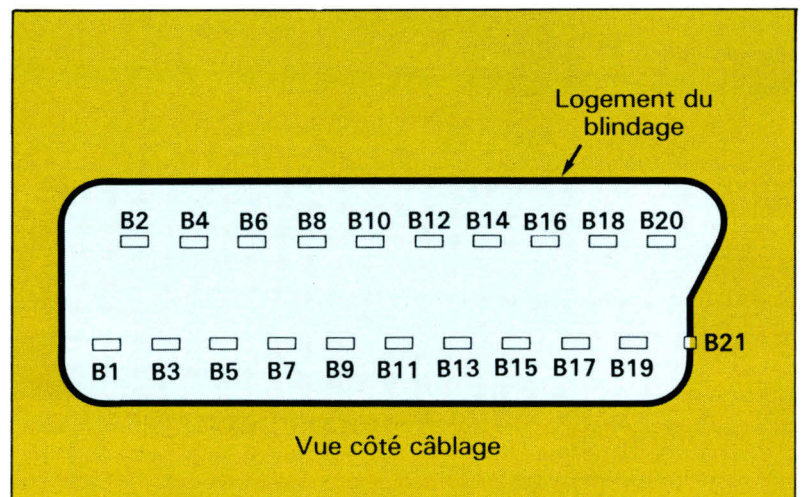
Fig. 3. – La prise Péritel : identification des contacts de l'embase, vue du côté câblage.
