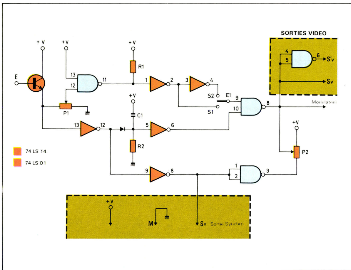
Fig. 1. - Schéma de « l'inverseur vidéo » légèrement modifié pour permettre la connexion avec notre montage : seul un inverseur supplémentaire est utilisé.
