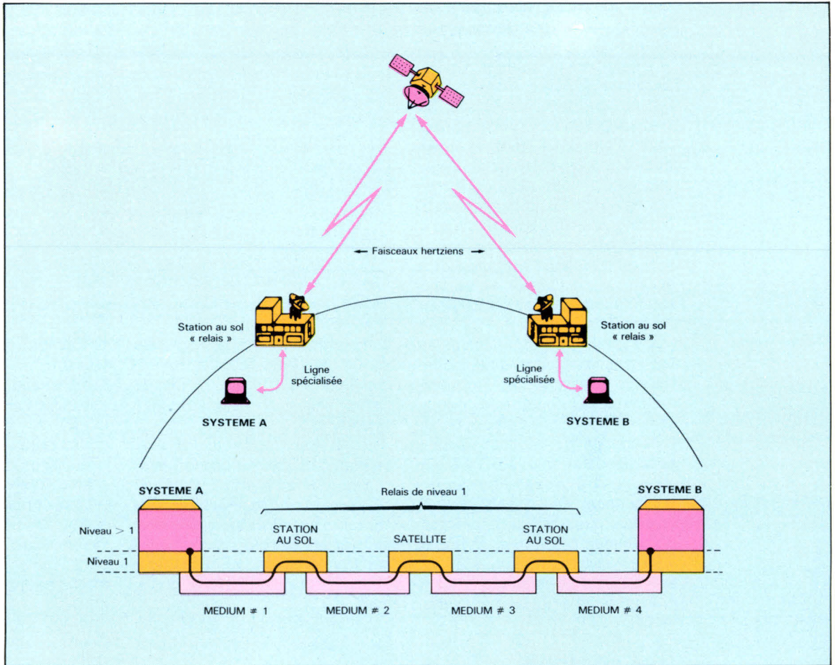
Fig. 4. – Représentation schématique d'une liaison par satellite (selon le modèle de l'ISO).
