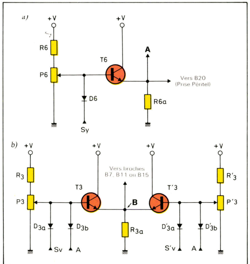
Fig. 2. - a) « Amplificateur simple » délivrant un signal de « synchro » aux exigences de l'entrée Péritel. - b) « Amplificateur double ». Il permet d'obtenir une composante fondamentale de couleur. Deux autres « amplificateurs doubles » identiques sont nécessaires.
