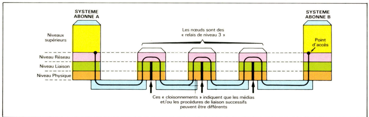
Fig. 7. - L'élément de réseau représenté selon notre modèle.
