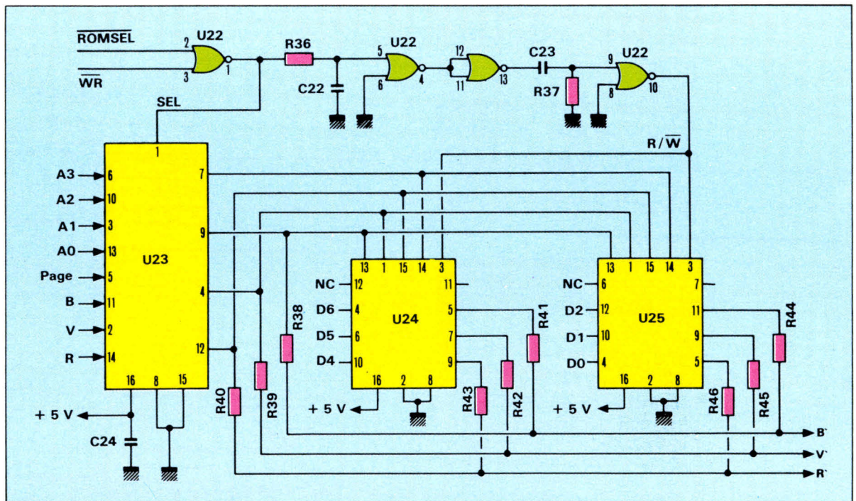
Fig. 2. - Schéma de principe de la carte.
