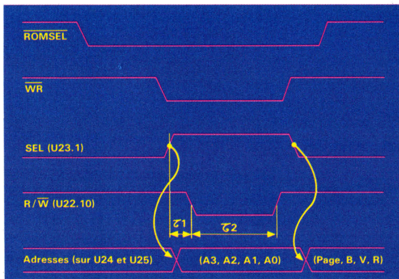
Fig. 3. - Ecriture dans la mémoire de la palette par le Z-80.
