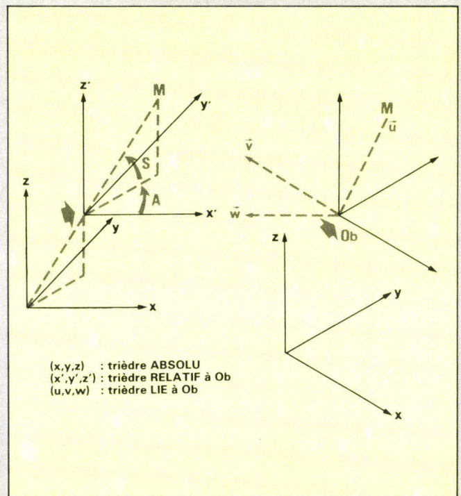
Visualisation du changement de repère correspondant à la position de l'observateur (ce dernier n'étant pas nécessairement à l'origine de l'espace de définition de l'objet).
