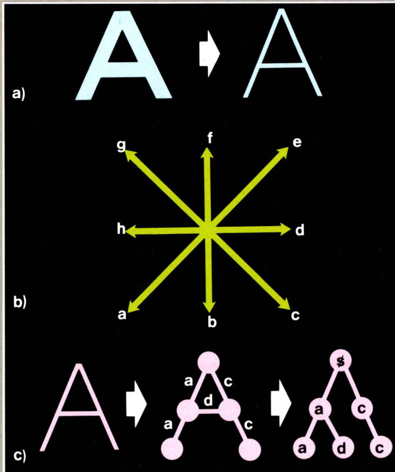
Fig. 9. – Représentation de caractères. a) La squelettisation supprime la redondance d'un caractère et réduit sa forme à quelques segments symboliques. b) La direction de chaque segment est déterminée selon le code de Freeman. c) A chaque segment est attribué un code (a, b, c, ..., h) correspondant à sa direction. Le caractère est ensuite développé en arbre, partant du sommet en haut et à gauche, auquel est affecté le nœud étiqueté $; les autres nœuds sont obtenus à partir des autres sommets et des intersections du squelette.
