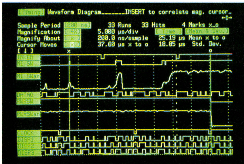
Visualisation simultanée des signaux logiques et analogiques.
