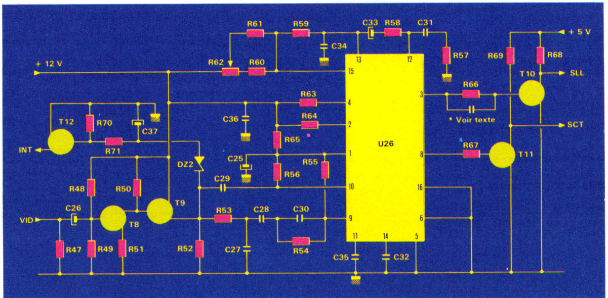
Fig. 8. - Schéma de principe du montage.
