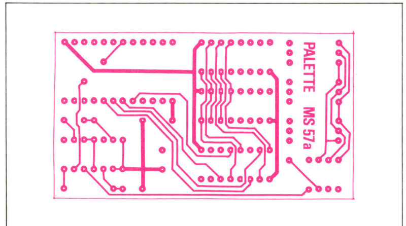
Fig. 4b - Circuit imprimé côté soudures.
