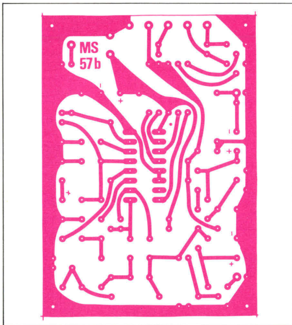
Fig. 9a. - Circuit imprimé côté soudure.
