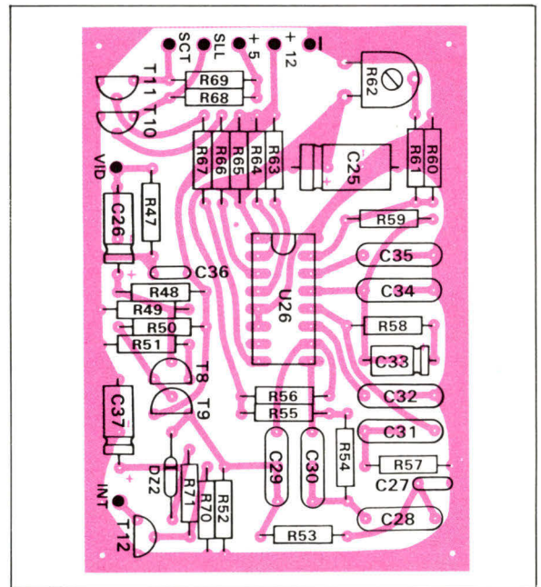
Fig. 9b. - Implantation des composants.
