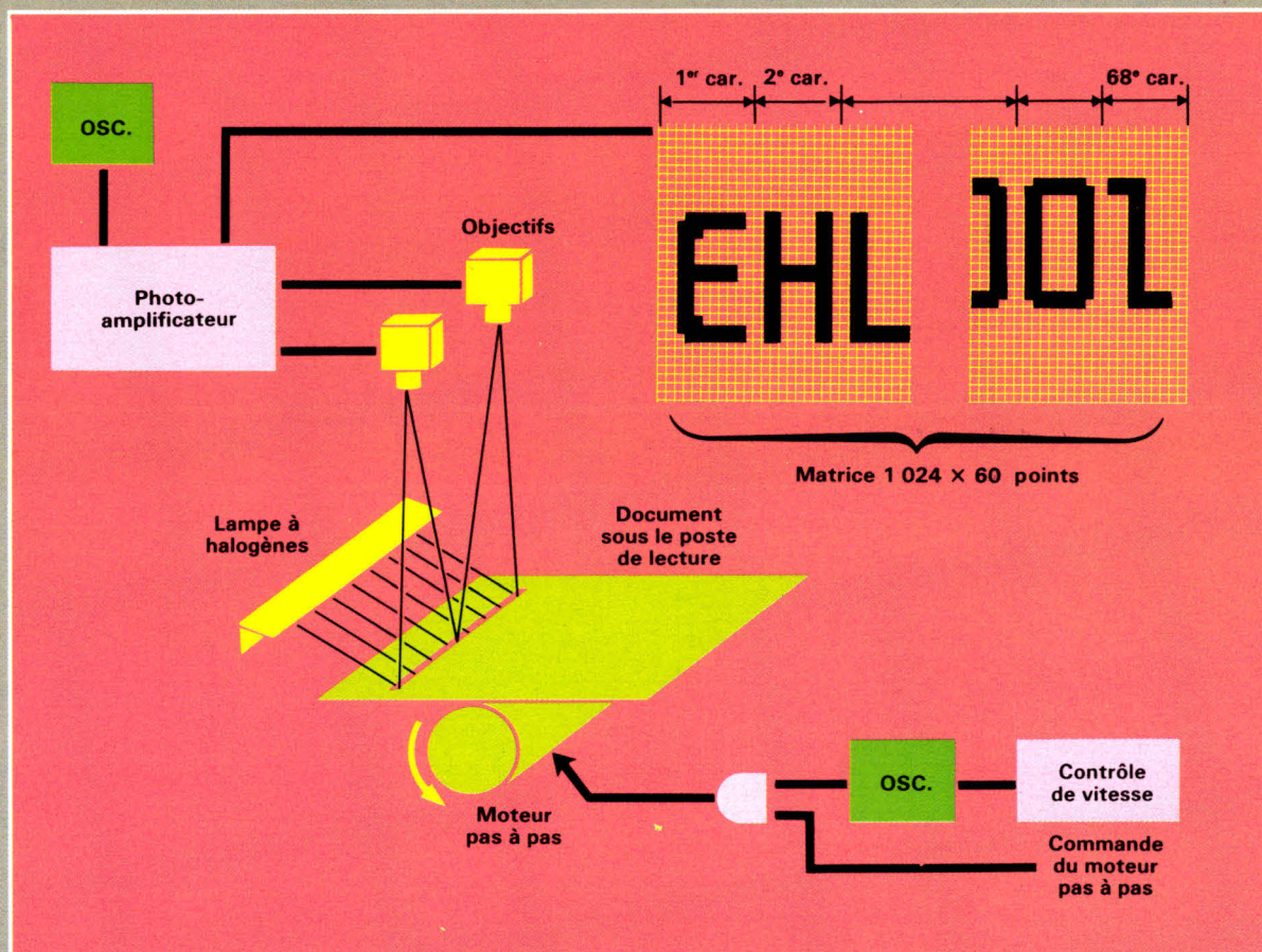
Fig. 3. - Saisie optique par une matrice de photodiodes (d'après doc. Feller).
