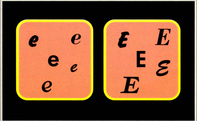
Fig. 7. - Exemple de partition d'un ensemble constitué de E majuscules et minuscules.
