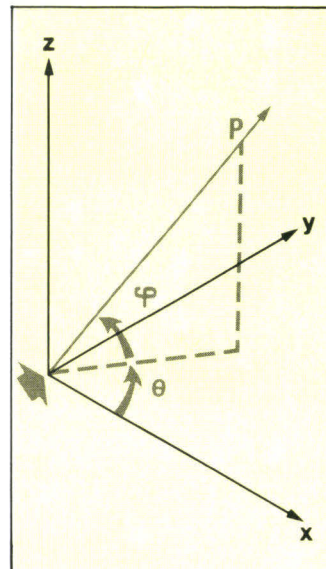
Fig. 2. - La direction d'une droite partant d'une origine est définie parfaitement par deux angles dits d'azimuts et de site.
