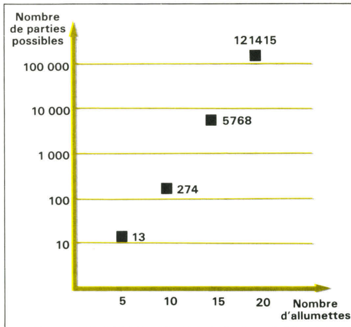
Fig. 2. — Indication sur une échelle semi-logarithmique du nombre de combinaisons possibles en fonction du nombre initial d'allumettes.
