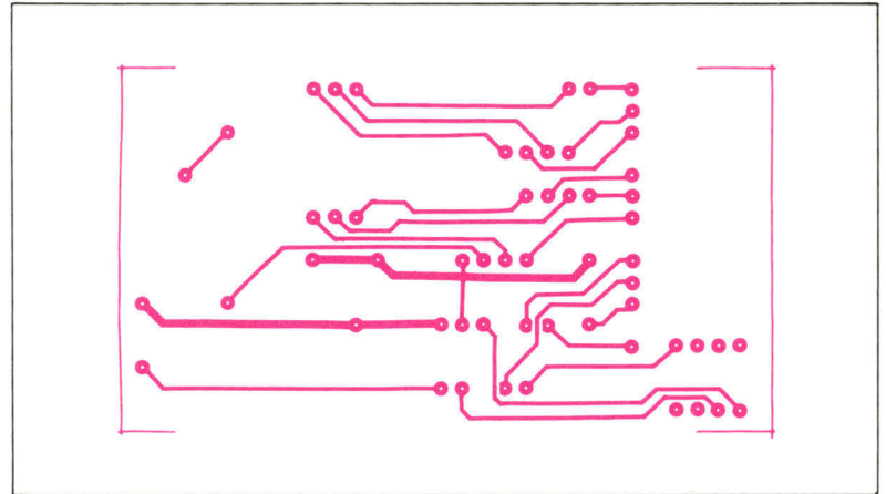
Fig. 4a. - Circuit imprimé côté composants.
