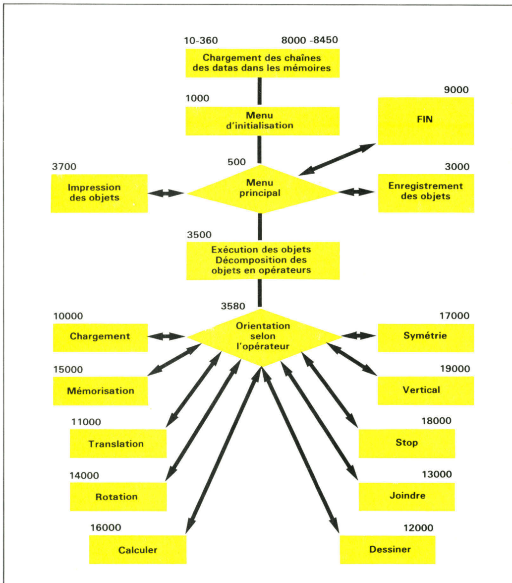
Fig. 11. – Organigramme de Mykérinos.
