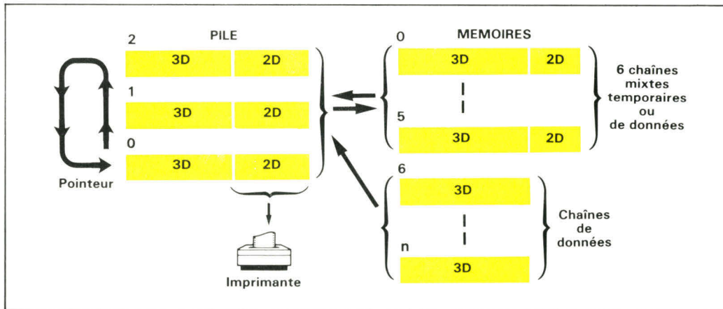
Fig. 10. – Structure de fonctionnement de la pile et de la gestion mémoire de Mykérinos.
