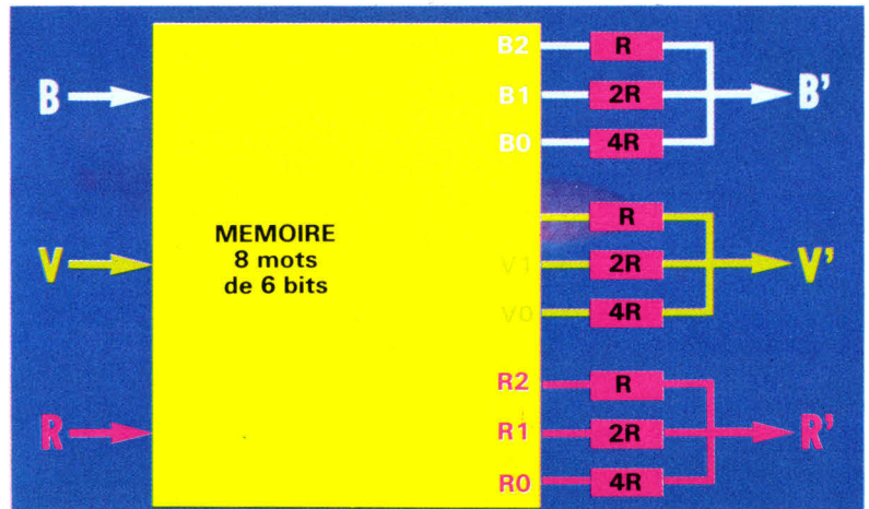
Fig. 1. - Principe de fonctionnement de la palette de couleurs.
