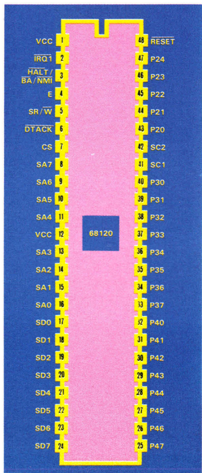
Brochage du MC 68120.
