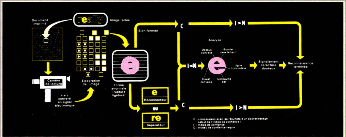
Fig. 5 - Identification des caractères par le lecteur KDEM (d'après doc. Kurzweil).
