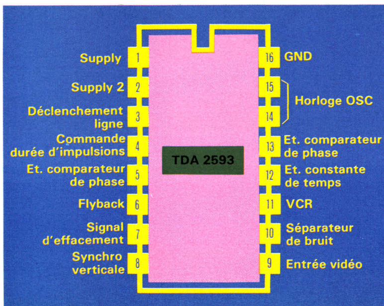
Fig. 7. - Brochage du TDA 2593.
