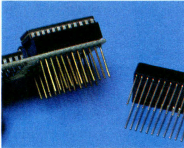
Un support à wrapper permet l'enfichage sur la carte de base.
