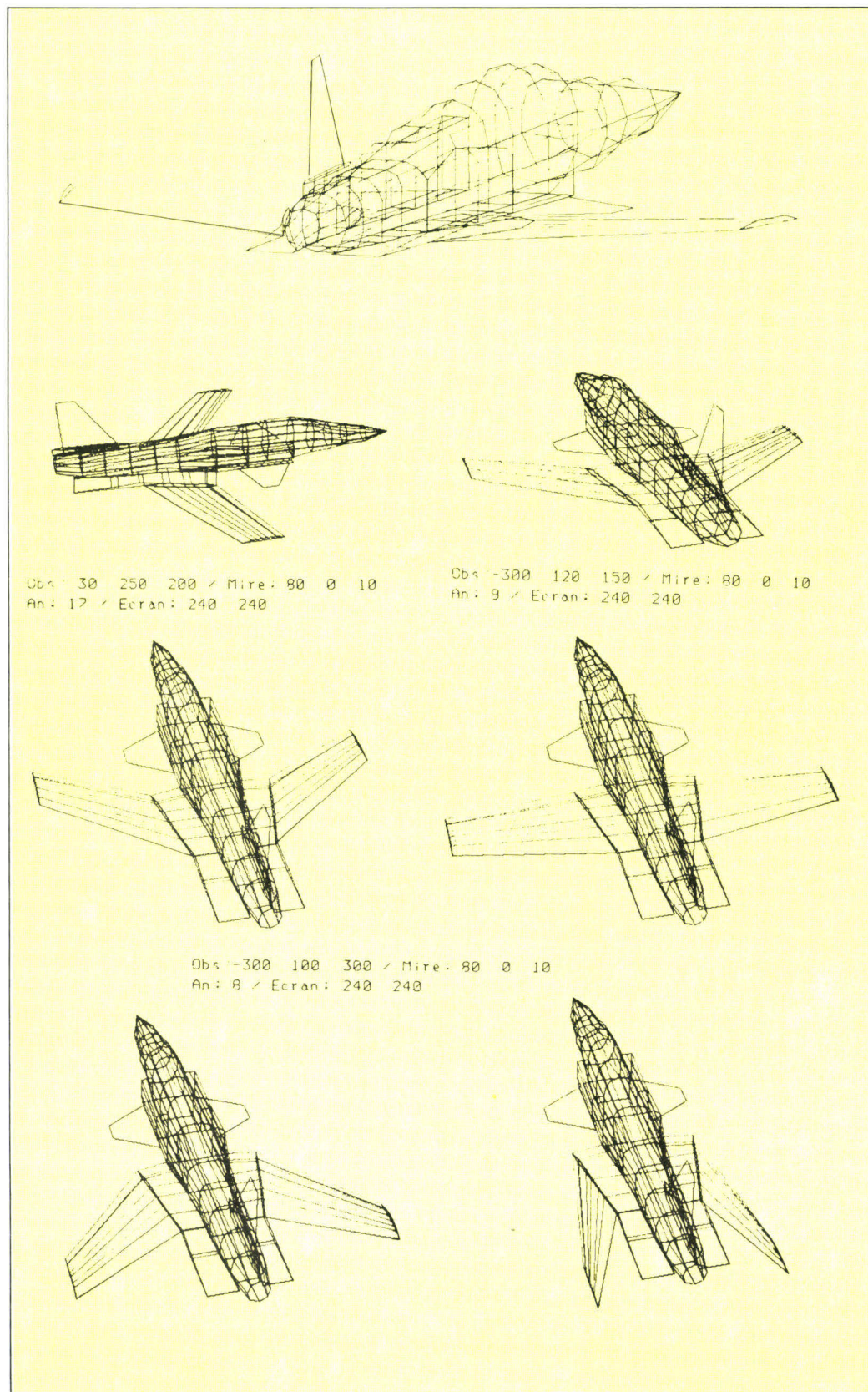
Fig. 8. - Dessin du prototype Grumman X-29 à l'aide de Mykérimos.
