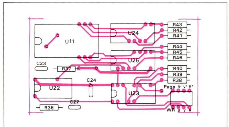
Fig. 4c. - Implantation des composants.
