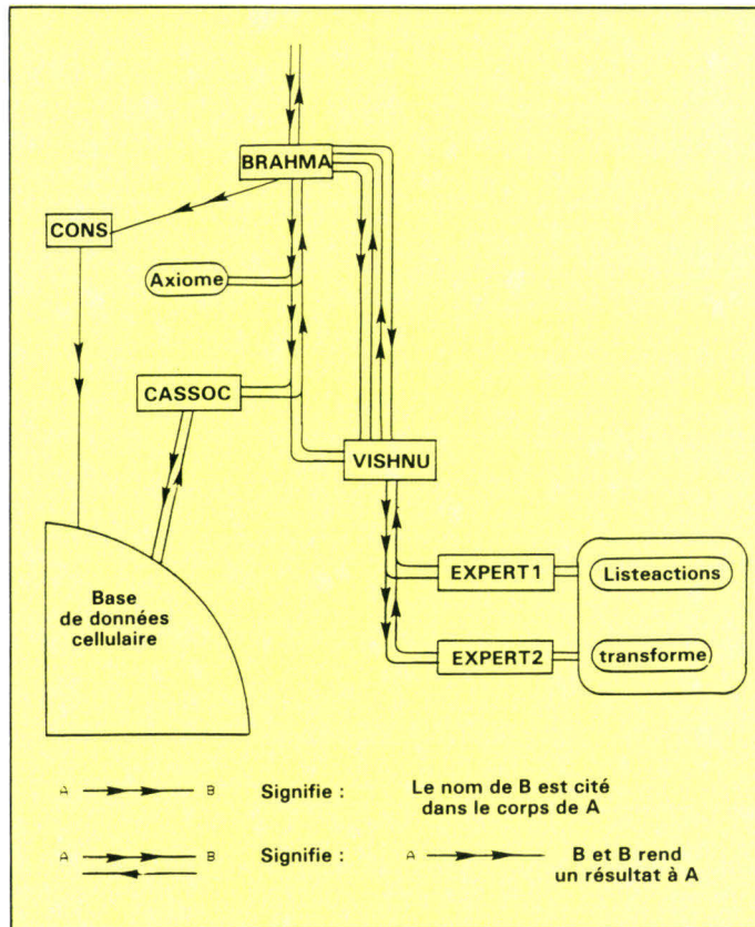
Fig. 3. - Circulation des informations dans le noyau du programme.
