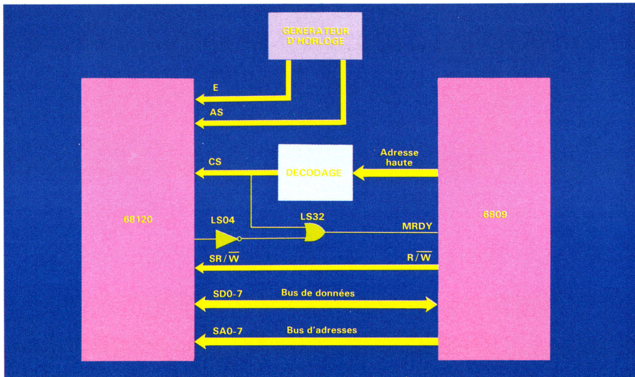
Schéma d'interconnexion type entre un 68120 et un 6809 de Motorola.
