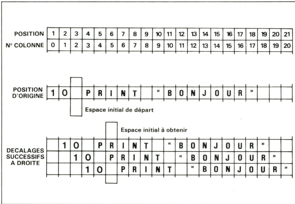
Fig. 3. - Exemple de déplacement de lignes par insertion d'espaces.
