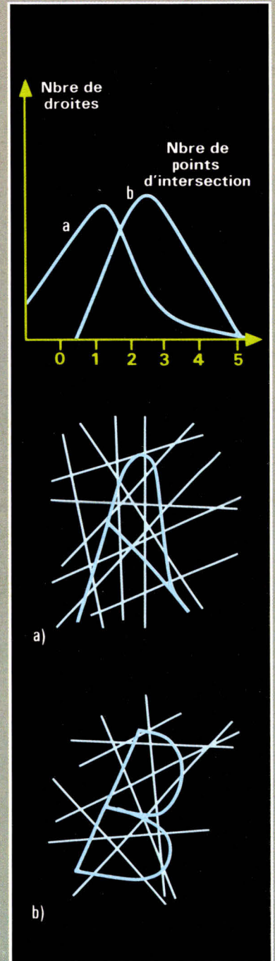
Fig. 10. – En reconnaissance des formes, certaines heuristiques, a priori curieuses, donnent d'excellents résultats. C'est le cas de la méthode des droites aléatoires pour reconnaître des caractères. Un certain nombre de droites aléatoires (environ 50) sont tracées : l'histogramme du nombre de droites ayant 1, 2, 3, ..., n points d'intersection avec la forme étudiée fournit un moyen de séparation pour quelques classes de lettres. C'est l'algorithme de Jung Pyo Hong (d'après G. Guilho et J.-P. Jouannaud, La Recherche n° 43, mars 1974).
