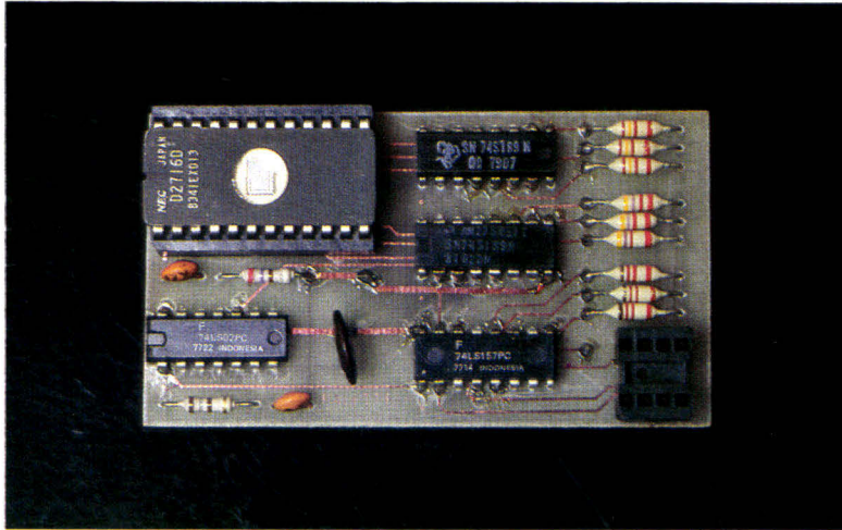
La carte palette de couleur reprend l'EPROM de la carte graphique de base.
