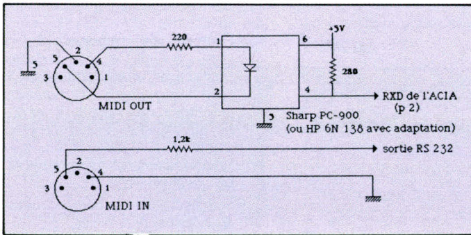
Fig. 7. - Adaptation des niveaux MIDI/RS 232.
