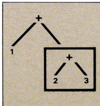
Fig. 1. - Arbre syntaxique de l'expression 1+2+3.
