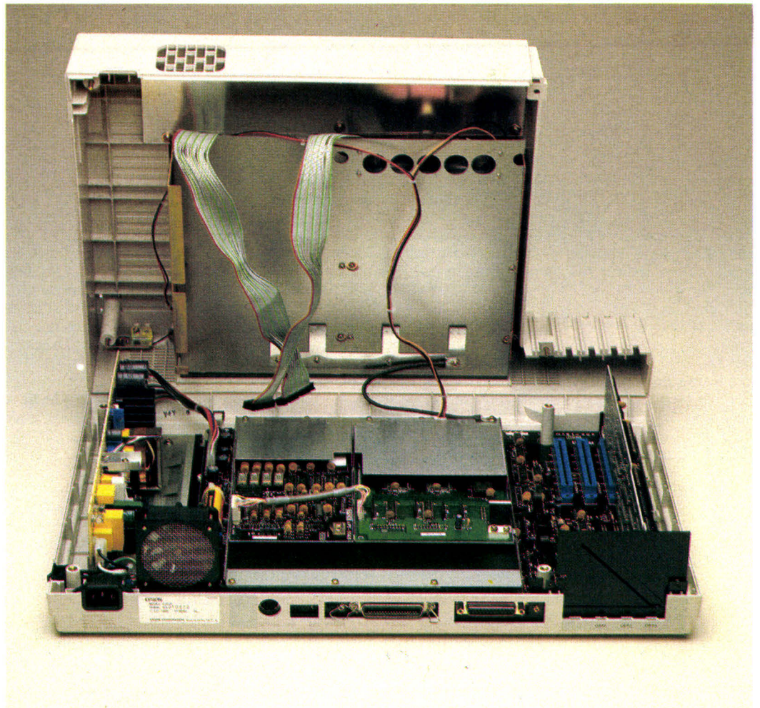
L'intérieur du QX 6 révèle 3 slots d'extension dont un (à droite) est déjà occupé.
