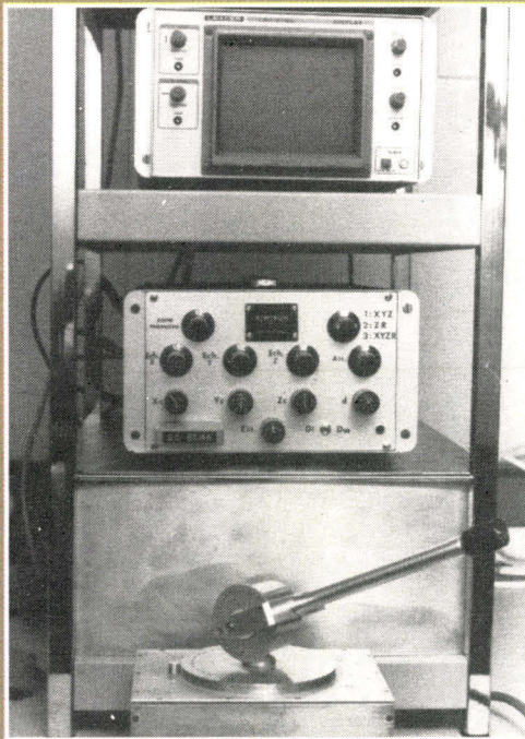
Calculateur analogique de perspective réalisé par le laboratoire de mécanique physique (Paris VI). A gauche, système minimal fonctionnant en autonomie. A droite, couplé à un micro-ordinateur et muni d'un moniteur de visualisation à grand écran.
