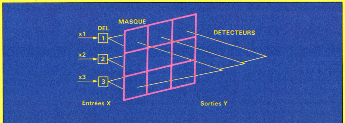
Fig. E. — La matrice est représentée par un masque. A chaque élément de matrice correspond une cellule du masque dont la transparence est fonction de la valeur de l'élément.
