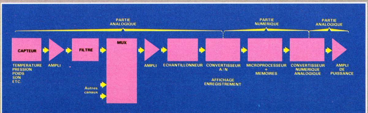
Fig. 4. – Système typique d'acquisition de données. (D'après doc. Intersil.)
