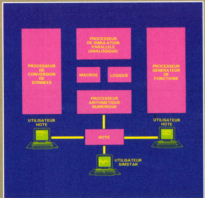
Fig. 8. – Organisation d'un calculateur hybride : Simstar (EAI).
