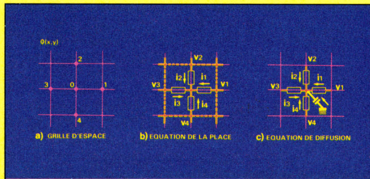
Fig. A. - A chaque point de la grille d'espace (xy) correspond un nœud du réseau électrique (a). La mesure des différents potentiels V(x,y) permet de résoudre soit l'équation de Laplace, dans le cas d'un réseau passif (b), soit l'équation de diffusion, avec un réseau actif (c).
