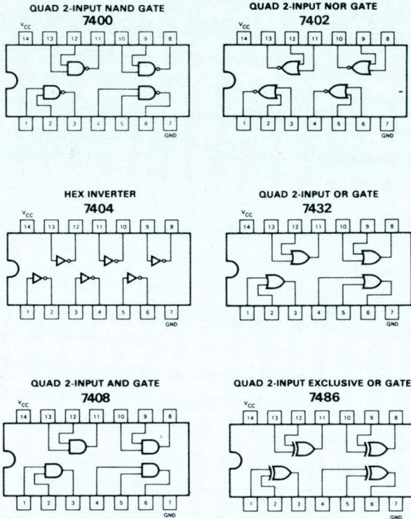
Fig. F. - Brochage des composants logiques employés pour cet article.
