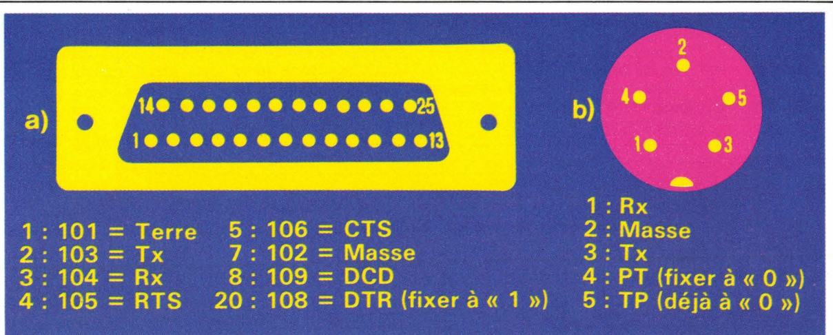
Fig. 5. – Brochage de la prise RS 232 C (a) et de la prise DIN minitel (b).
