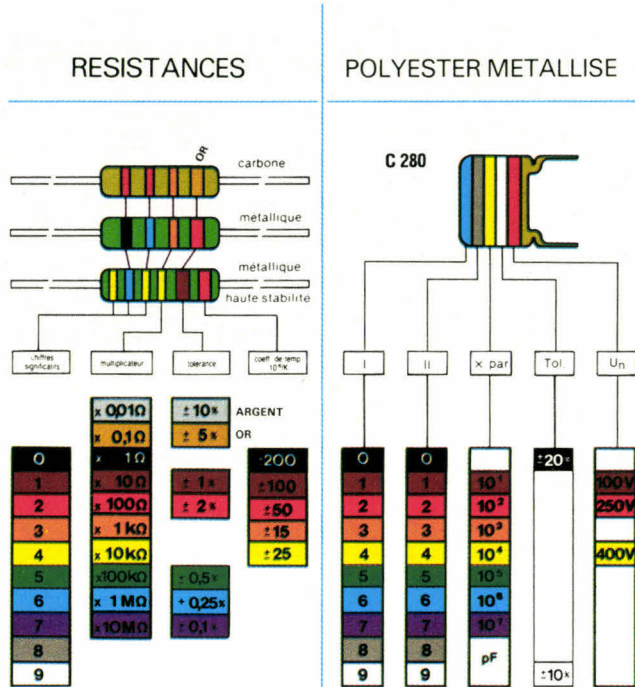
Fig. A. - Code des couleurs permettant de connaître valeur et tolérance d'une résistance.
