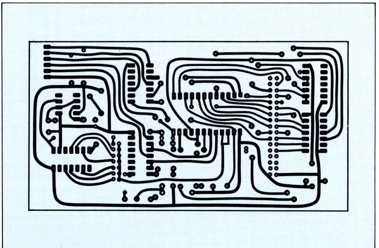
Fig. 4a. - Circuit imprimé côté cuivre.
