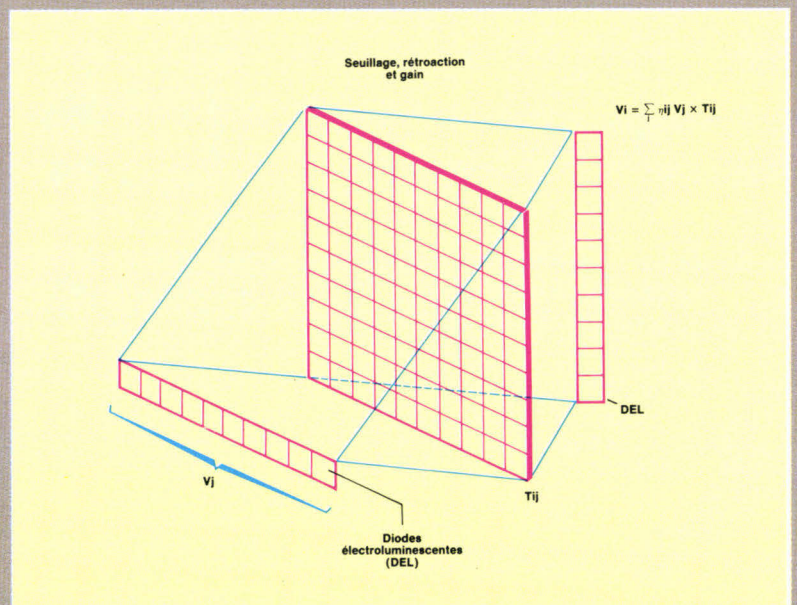
Fig. 8. – Le modèle de Hopfield peut être réalisé à partir de dispositifs optiques bistables comprenant un multiplicateur vecteur-matrice et un système de rétroaction non linéaire.
