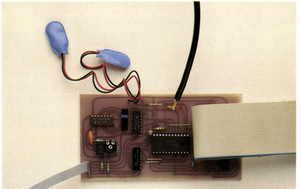
Fig. 6. – Programme n° 1.
