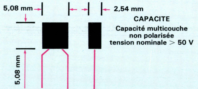
Fig. C. - Description des capacités multicouche non polarisées.
