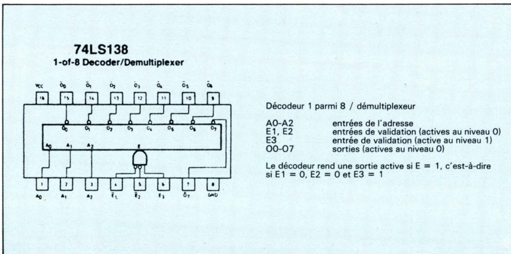
Fig. 15. - Brochage du décodeur 74LS138.
