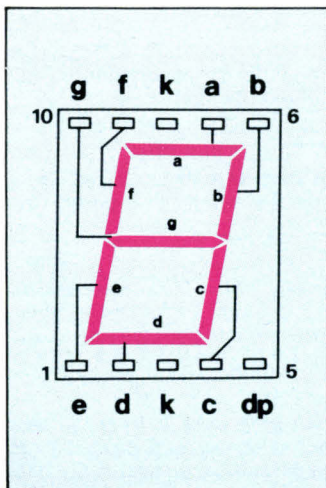
Fig. 8. – Schéma de brochage d'un afficheur 7 segments à cathode commune HDSP 5303.
