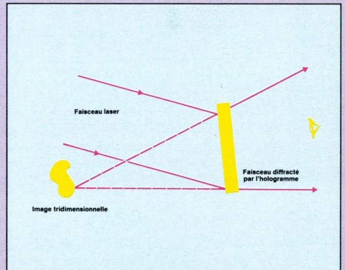
Fig. B. - Restitution de l'hologramme.
