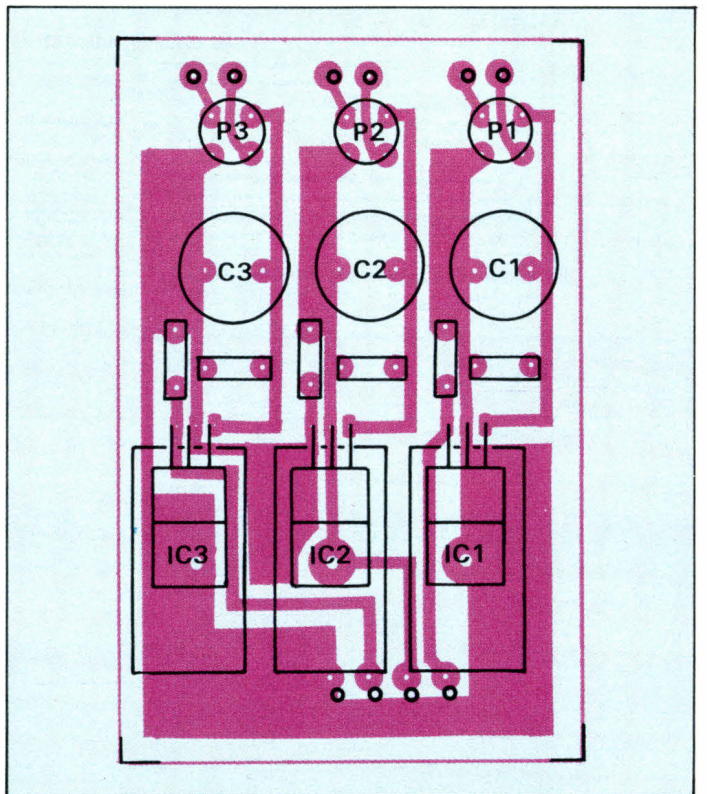
Fig. 8. - Implantation des composants de l'alimentation.
