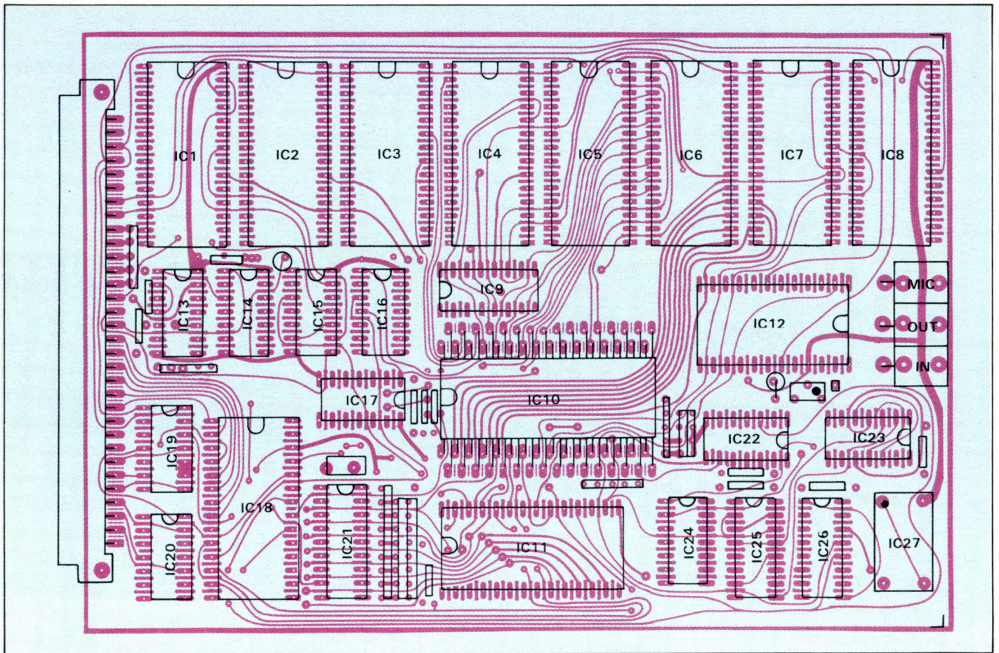
Fig. 3. - Implantation des composants de la carte reconnaissance.
