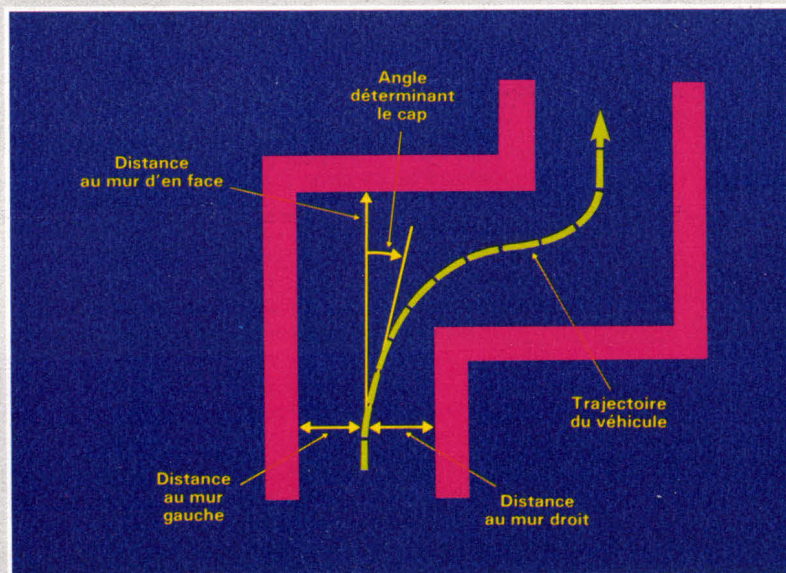
Fig. 10. - Un prototype de véhicule commandé par la logique floue se déplace à l'aide d'une vingtaine de règles fondées sur une combinaison du cap du véhicule et de sa distance aux murs bordant la chaussée. Le contrôleur ajuste le cap de la voiture afin de minimiser la différence entre les valeurs du cap et de la position spécifiées par les règles, et celles mesurées par un petit transducteur supersonique monté sur le véhicule.
