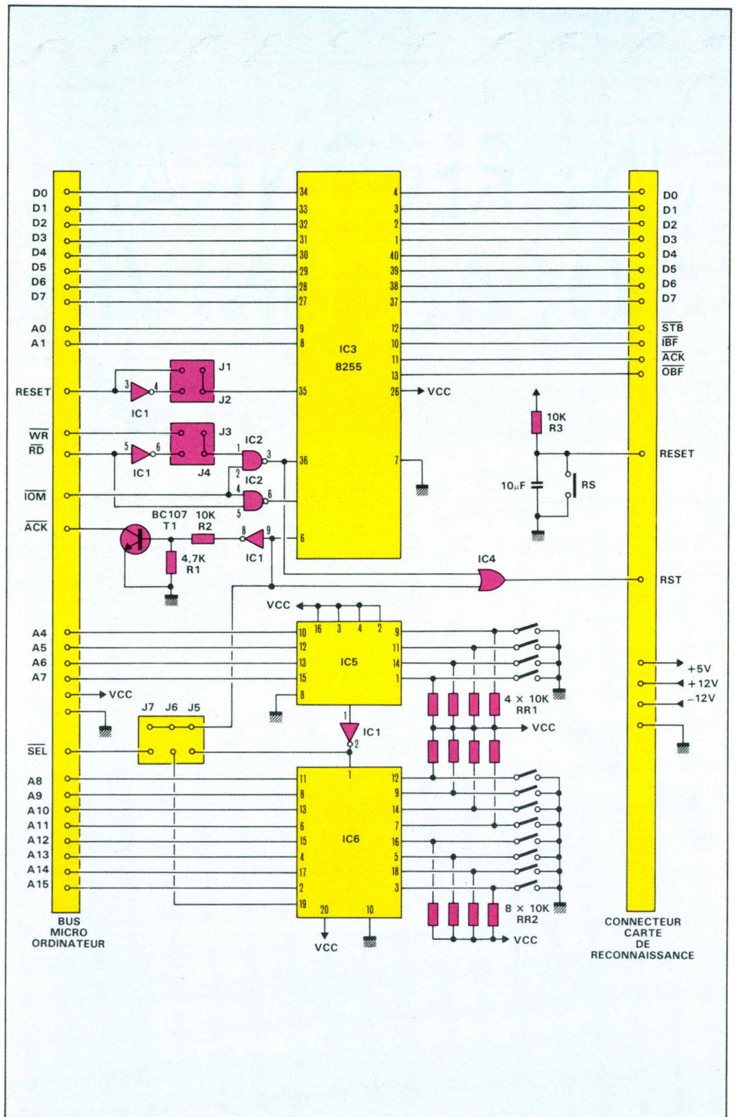
Fig. 1. - Schéma de principe de l'interface universelle.
