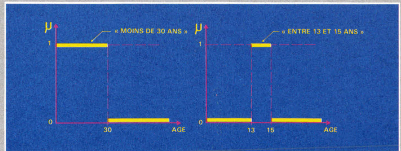
Fig. 3. - Fonctions d'appartenance correspondant aux concepts nets « MOINS DE 30 ANS » (a) et « ENTRE 13 ET 15 ANS » (b). Les fonctions sont constantes par paliers et ne peuvent prendre que les valeurs 0 et 1 ; entre ces paliers, elles présentent des discontinuités.
