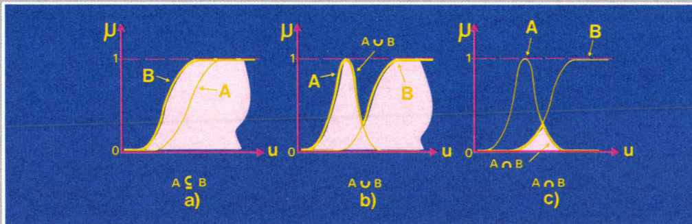
Fig. 6. – Fonctions d'appartenance correspondant à l'inclusion (implication), l'union (disjonction « OU ») et l'intersection (conjonction « ET ») d'ensembles flous : A \subseteq B : \mu_A(u) \leq \mu_B(u) \mu_{A \cup B}(u) = \max(\mu_A(u), \mu_B(u)) = \mu_A(u) \vee \mu_B(u) \mu_{A \cap B}(u) = \min(\mu_A(u), \mu_B(u)) = \mu_A(u) \wedge \mu_B(u)
