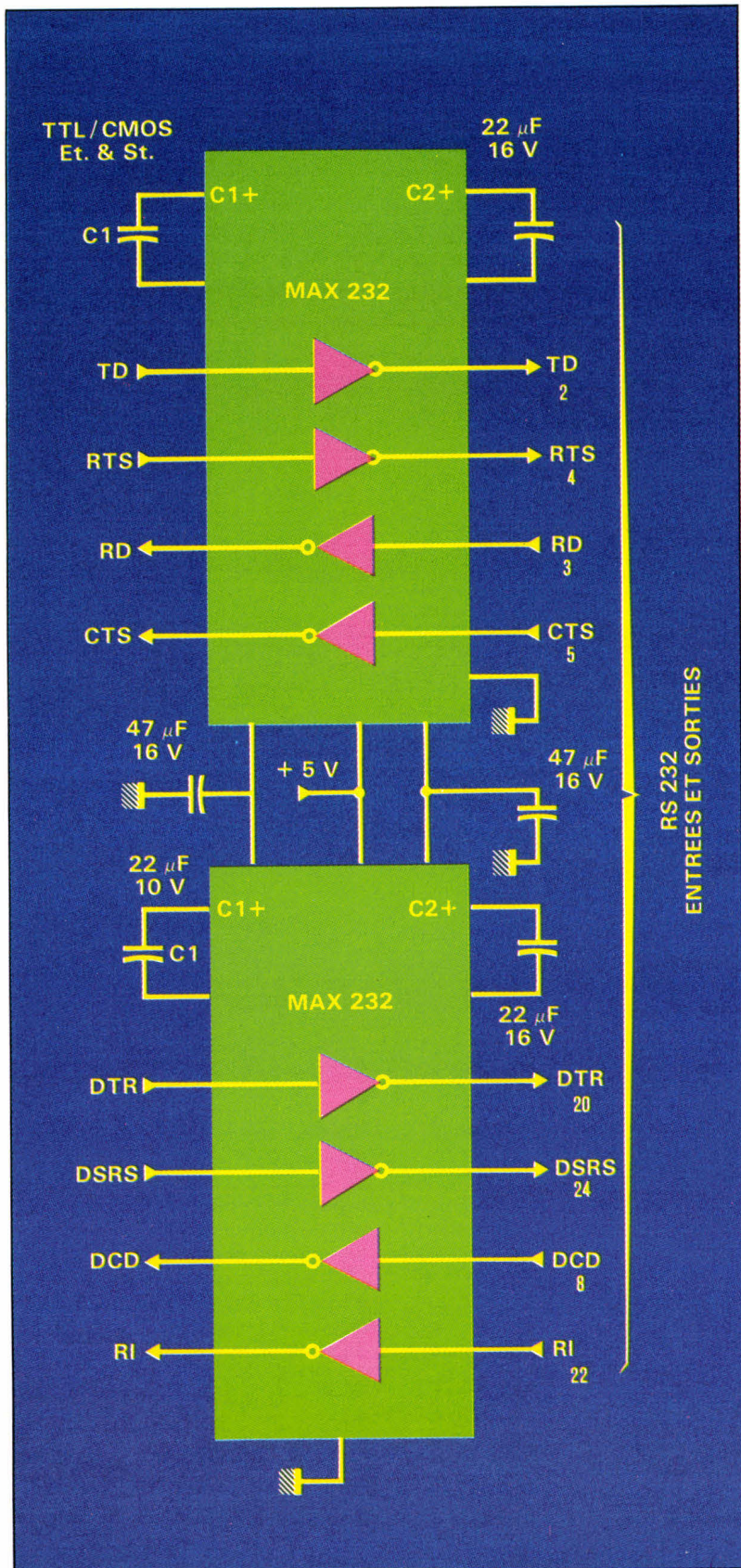
Combinaison de 2 MAX RS 232 pour 4 entrées/sorties.
