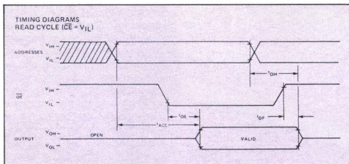
Fig. 4. - La mémoire morte.
