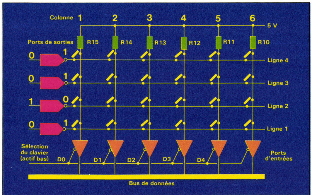
Fig. 1. - Schéma logique du clavier.
