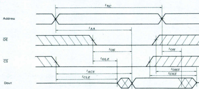
Fig. 10. - Caractéristiques temporelles de la 6116.
