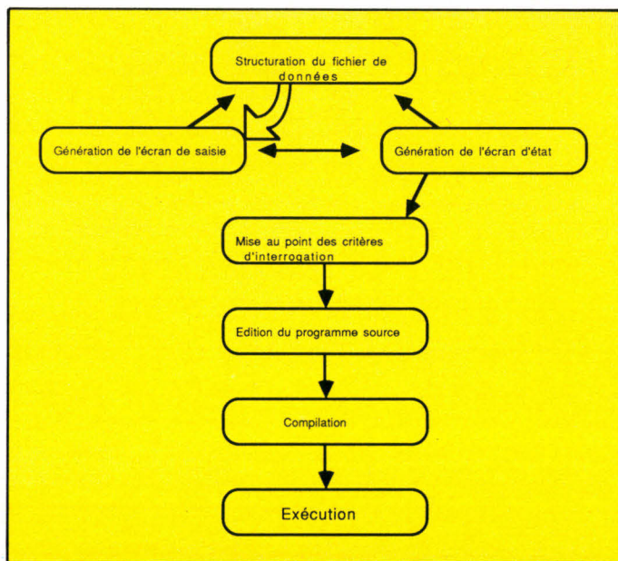
Fig. 1. - Etapes suivies pour la réalisation d'un programme Sublime.
