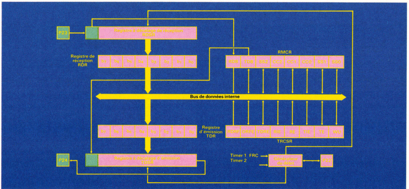
Fig. 8 - Interface de communication série.
