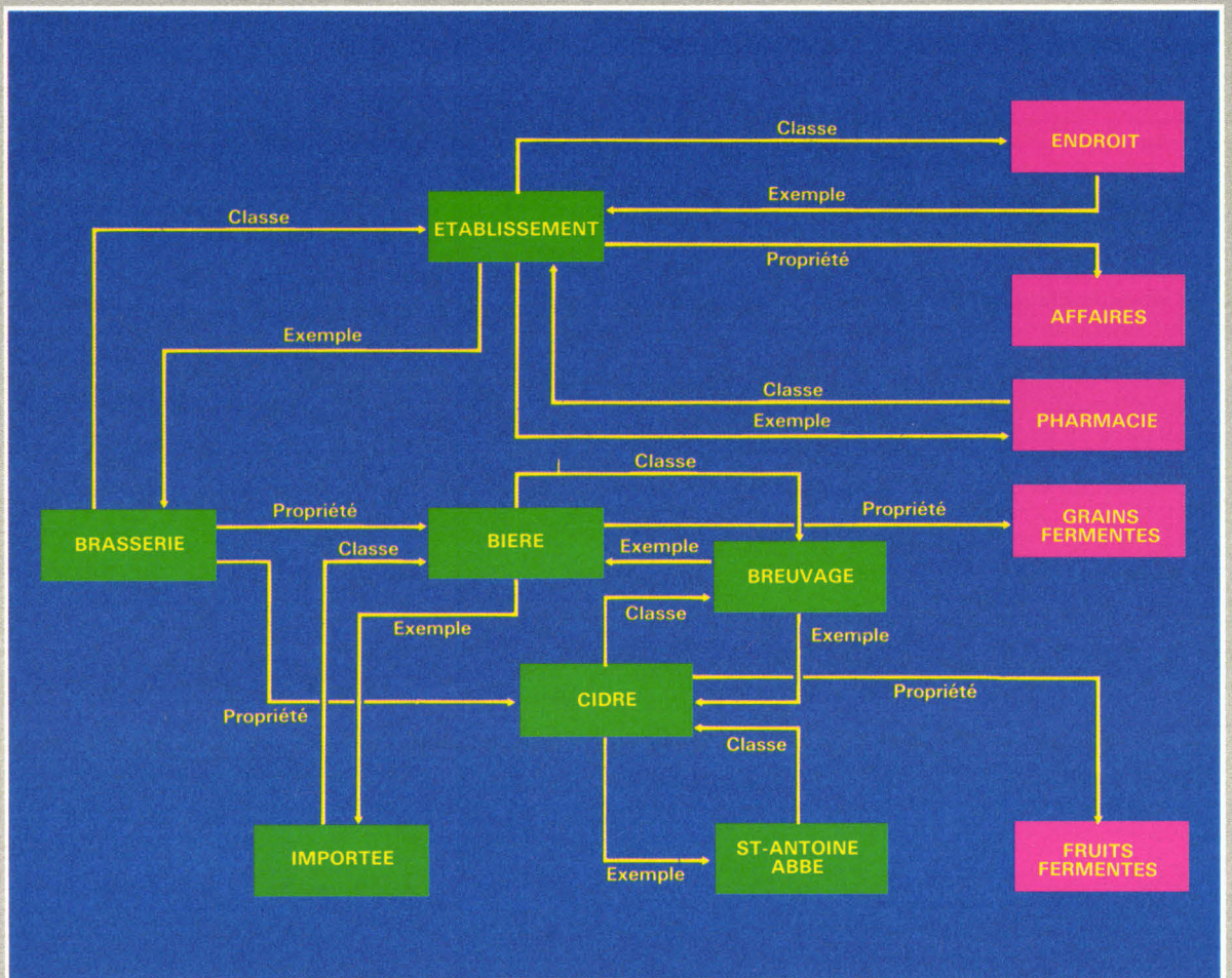
Fig. 8 - Un réseau sémantique peut être représenté graphiquement. Sous cette forme, il est plus facile à utiliser : un tel diagramme fait ressortir l'ensemble des interconnexions entre les composantes significatives (sémantiques) en mémoire. (D'après P. Roi).
