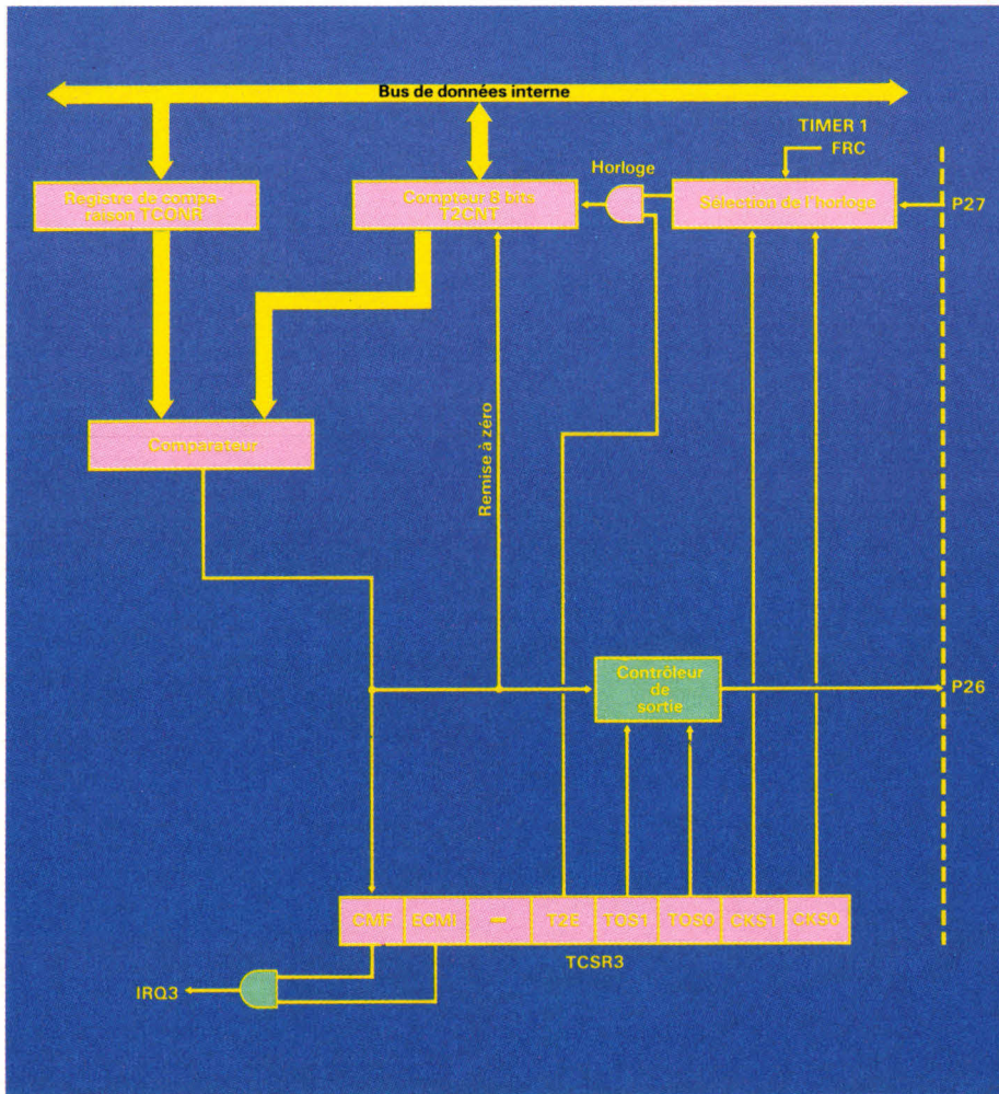
Fig. 7. - Timer 2.
