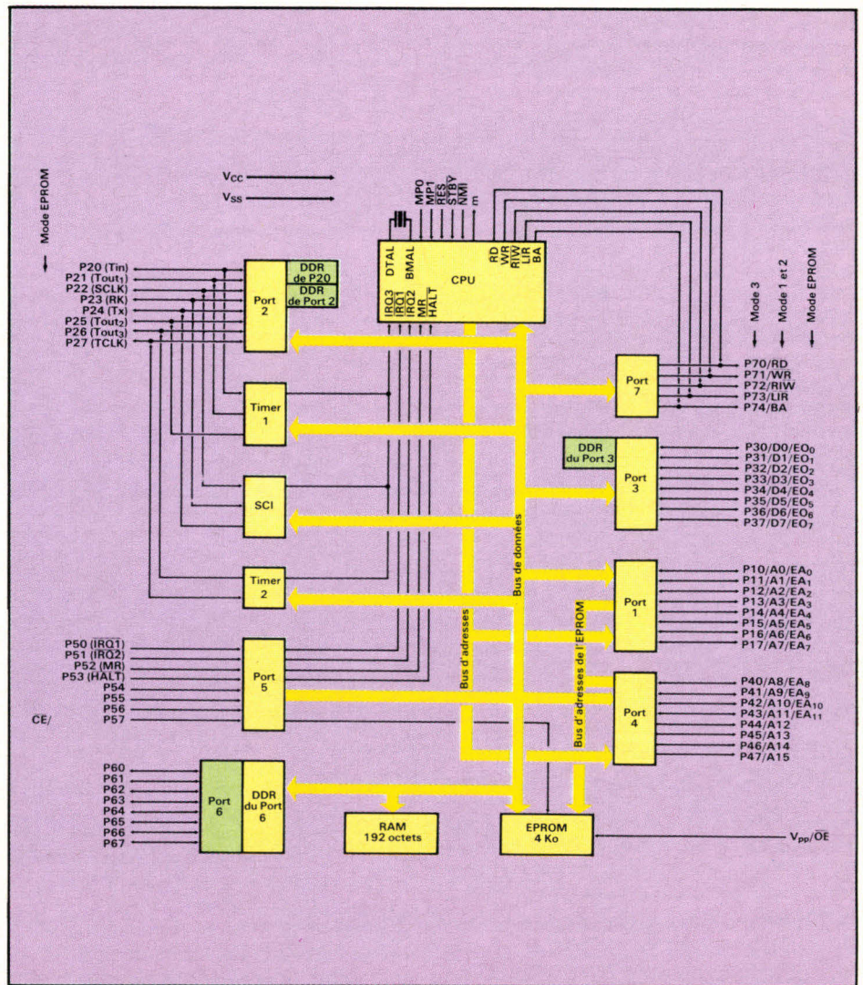
Fig. 1. - Le microcontrôleur HD 63701 XOC.
