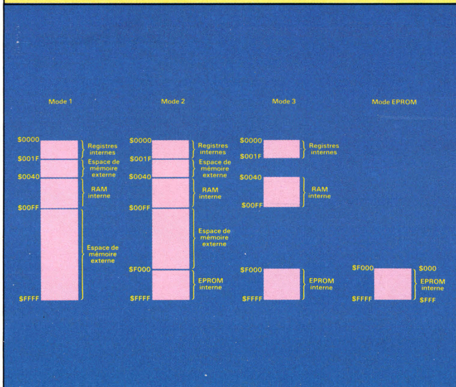
Fig. 3 - Carte mémoire.
