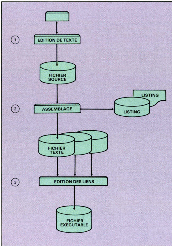
Fig. 1. - Procédure de développement en Assembleur.
