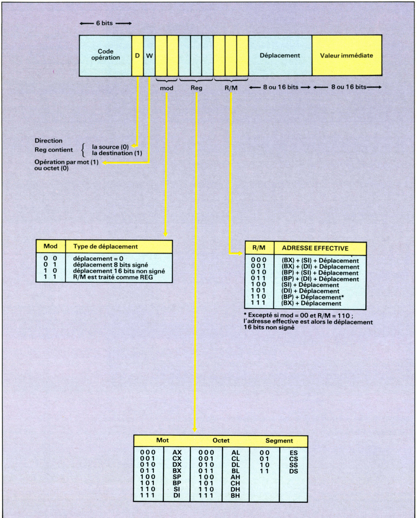
Fig. 3. - Format des instructions.
