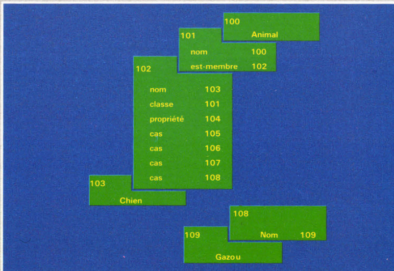
Fig. 7. - Dans un réseau sémantique, les concepts peuvent être rangés dans des registres de mémoire. Chaque concept est, à son tour, rattaché à un registre de mémoire : ainsi, le concept « animal » (registre *100) fait référence, via la relation « est membre » (*102), aux registres *103, *101, *104, etc. (D'après P. Roi).
