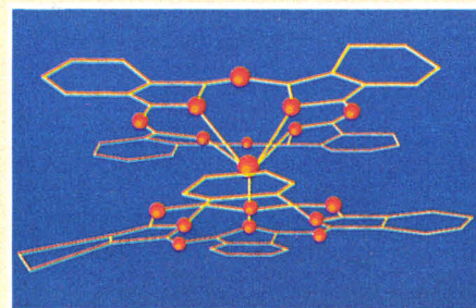
Fig. 5. — Molécule de diphtalocyanine de lutécium (PcLu) vue en plan (a) et de profil (b). L'atome de lutécium est visible entre deux groupements phtalocyanine. (D'après J. Simon.)
