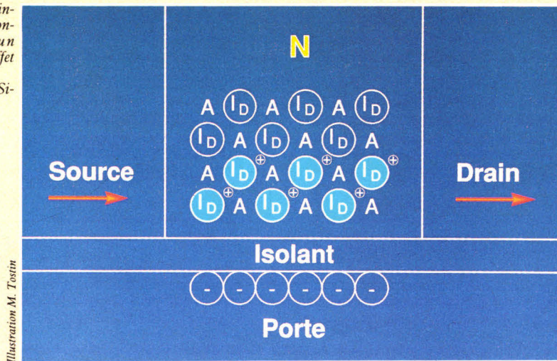
Fig. 7. - Transistor à effet de champ constitué d'une couche mince de phtalocyanine de zinc (PcZn) et diphtalocyanine de lutécium (Pc 2 Lu), déposées sur silice et silicium de type n. Les électrodes (drain et source) sont en or. (D'après J. Simon.)
