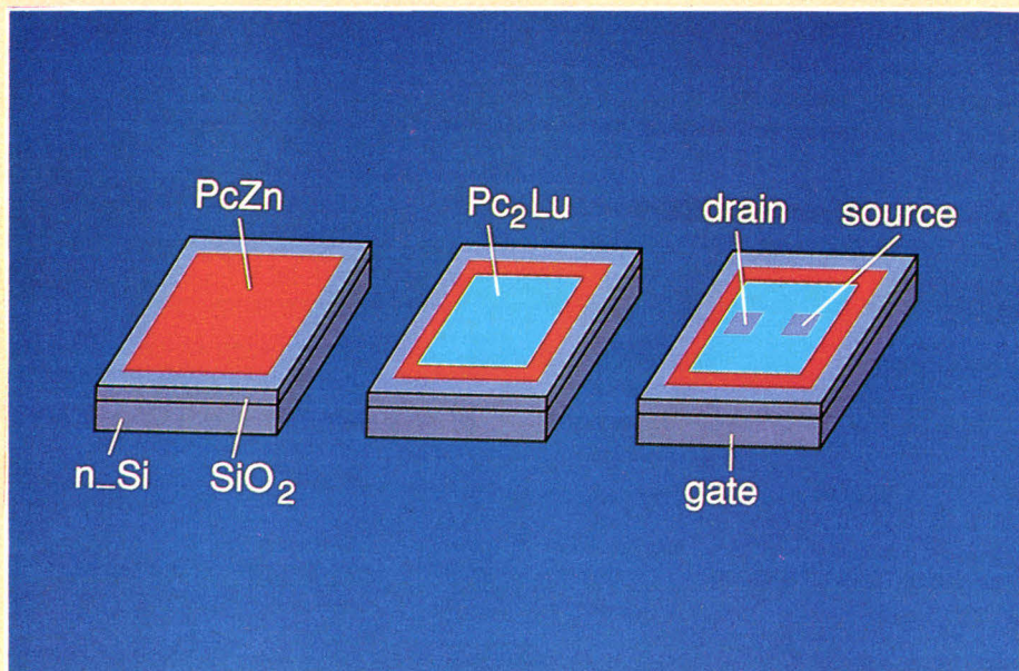
Fig. 7. - Transistor à effet de champ constitué d'une couche mince de phtalocyanine de zinc (PcZn) et diphtalocyanine de lutécium (Pc 2 Lu), déposées sur silice et silicium de type n. Les électrodes (drain et source) sont en or. (D'après J. Simon.)
