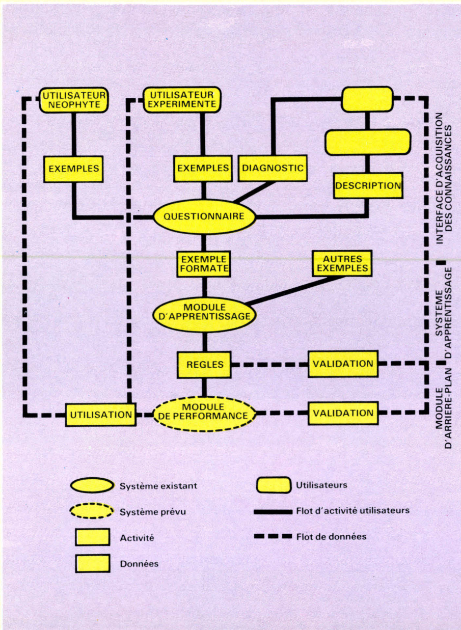
Fig. 2. – Constitution d'un système expert par apprentissage, dans le cadre de INSTIL (Integration of Numeric and Symbolic Techniques in Learning), à l'aide d'un questionnaire entre l'utilisateur (ou l'expert) et le système. (D'après doc. Cognitech.)
