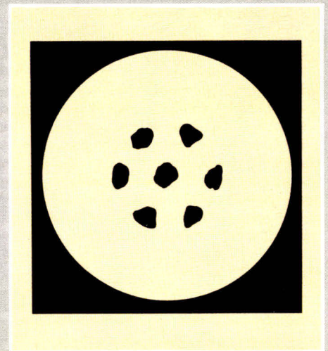
Fig. 5. — Coupe d'un fil à sept filaments. Diamètre du fil : 0,25 mm ; diamètre d'un filament ; 25 \mu\text{m} ; longueurs unitaires : quelques centaines de mètres. (D'après doc. CGE).
