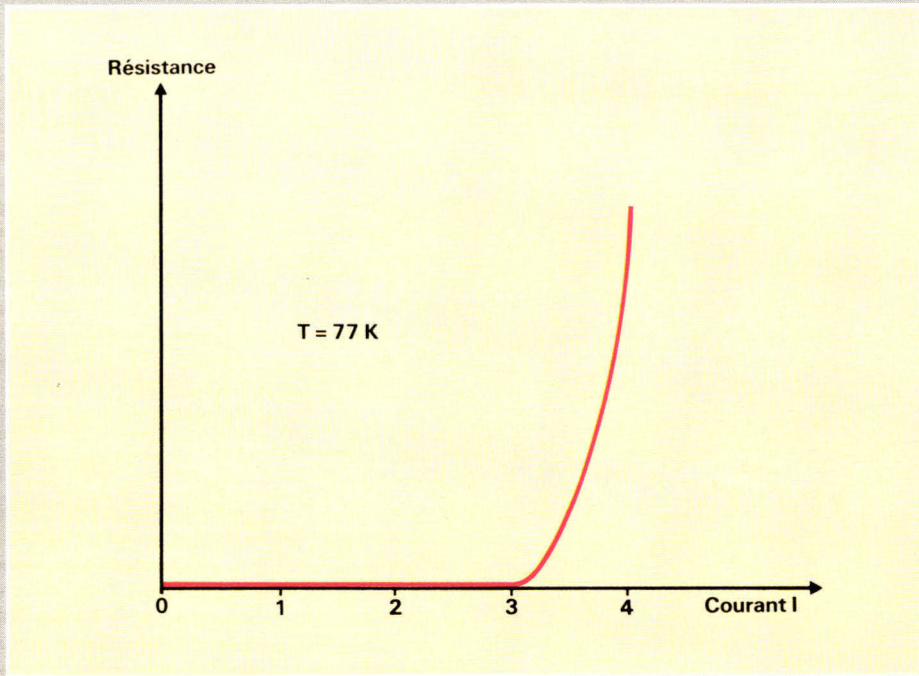
Fig. 3. — Transition résistive de YBaCuO. (D'après doc. CGE).
