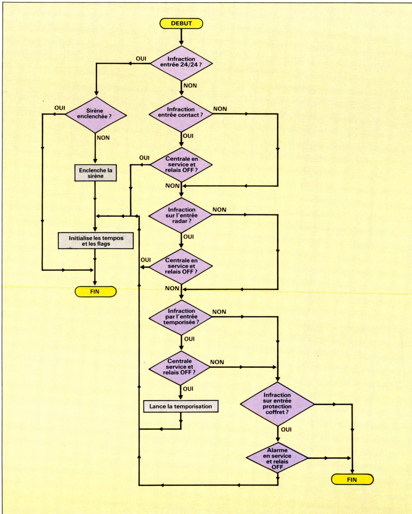
Fig. 3. – Organigramme du programme de lecture des entrées d'alarme.
