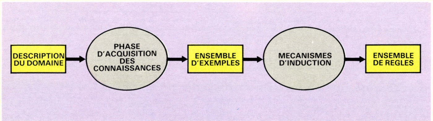
Fig. 1. – Processus automatique de construction d'une base de connaissances par apprentissage à partir d'exemples. (D'après doc. Cognitech.)
