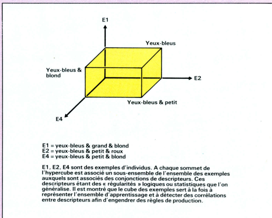
Fig. C. — Relations entre exemples et descripteurs dans Charade.
