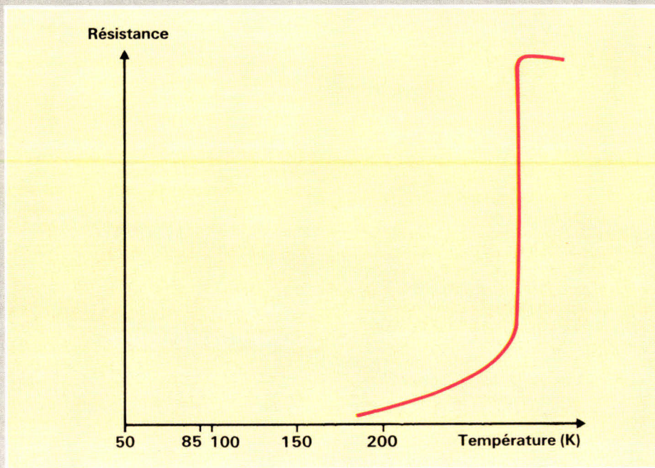
Fig. 4. — Courant en champ nul d'une pastille de YBaCuO. (D'après doc. CGE).
