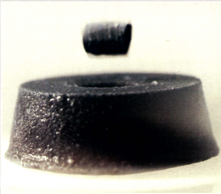
Expérience de lévitation d'un aimant céramique BaFe_{12}O_{19} au-dessus d'un tore céramique supraconducteur YBa_2Cu_3O_7 .
