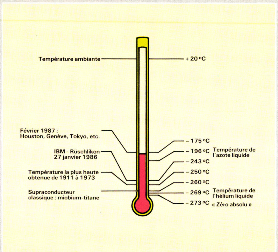
Fig 1. — La course aux températures critiques. (D'après R. Lavergne).
