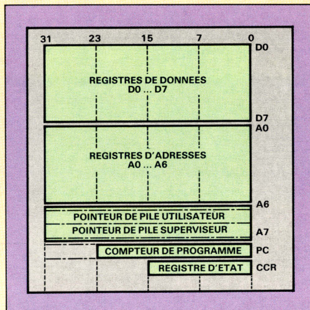
Configuration interne.
