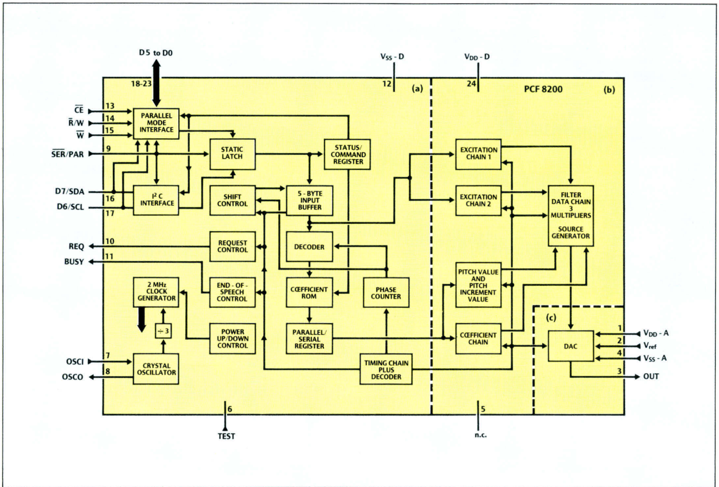
Fig. 1. – Schéma bloc du PCF 8200 – a) contrôle et interface microprocesseur – b) synthétiseur à formants – c) étage de sortie.
