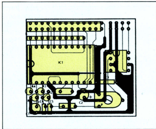
Fig. 9. Implantation des composants
