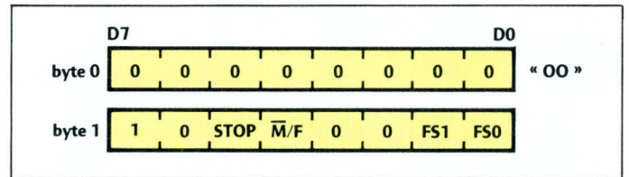
Fig. 2. – Format de la séquence de contrôle.
