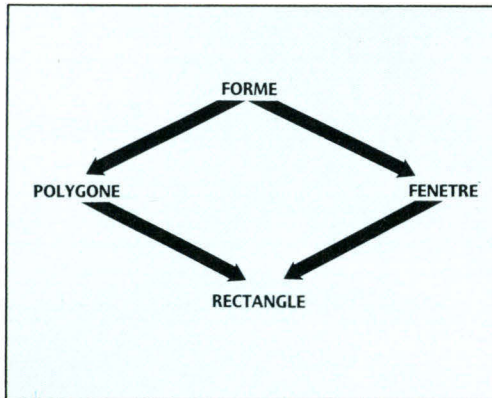
Fig. 3. – En cas de conflit d'héritage (valeurs ou méthodes venant de deux pères différents), deux stratégies de résolution peuvent être exploitées. Sur le chemin de priorité gauche (polygone - fenêtre - forme). Flavors choisit le premier élément et Loops conserve le dernier.
