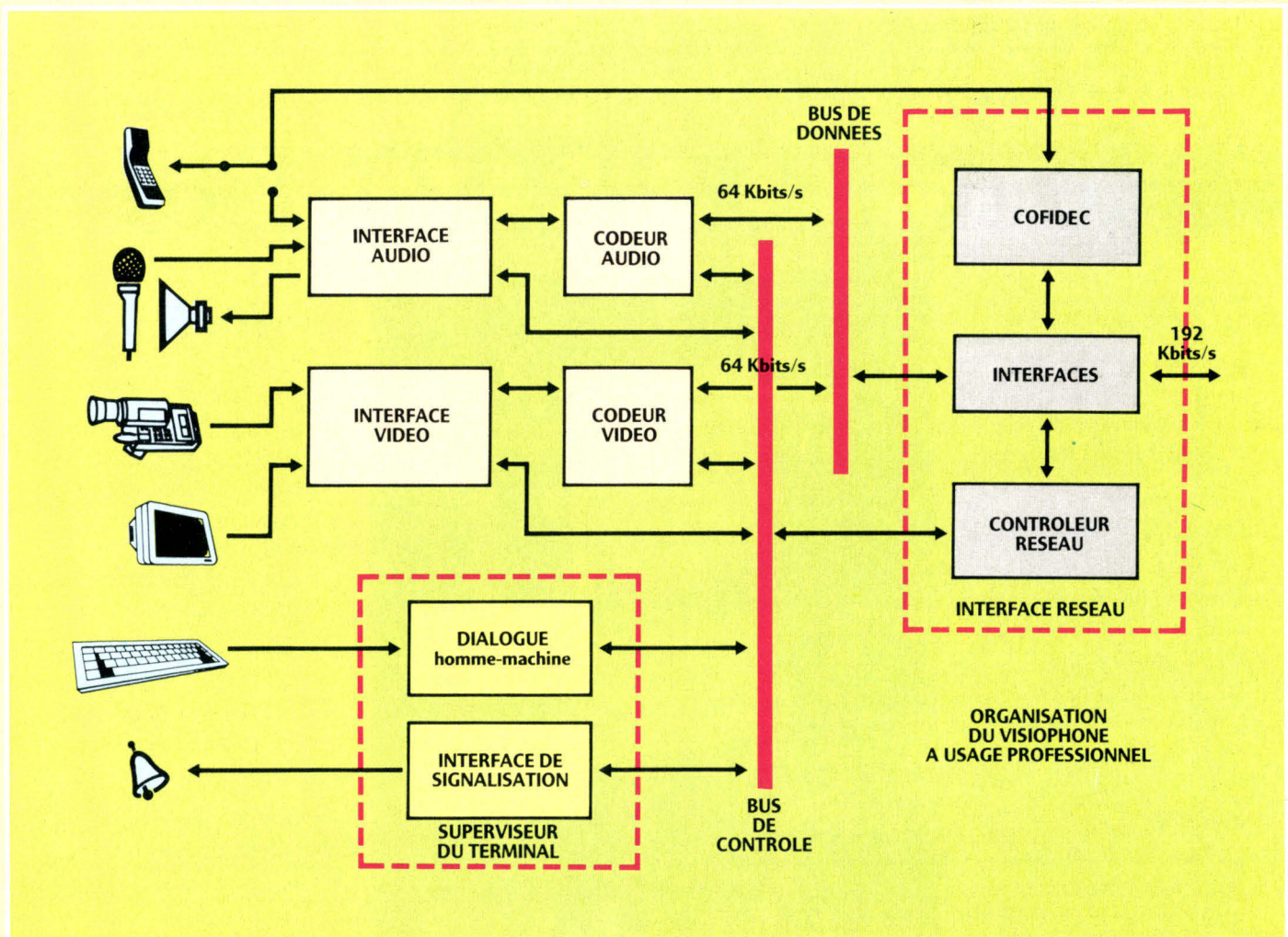
Fig. 8. – Organisation du visiophone professionnel.
