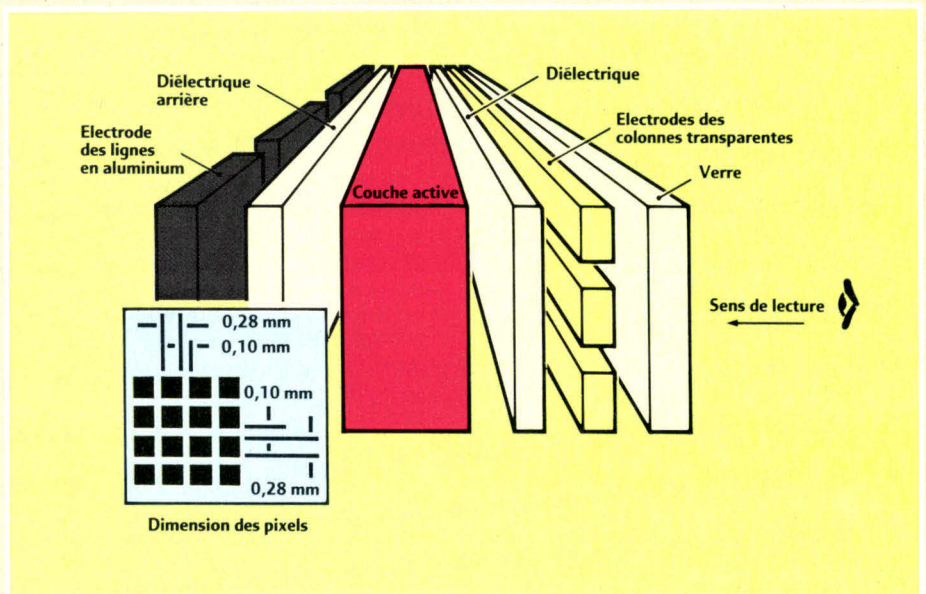
Fig. 3. - Structure des écrans électroluminescents (document Sigmatron Nova/Magazine Opto n° 44).
