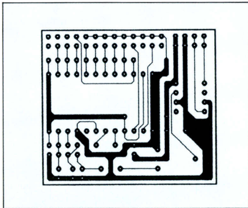
Fig. 8. - Circuit imprimé vu côté soudures.
