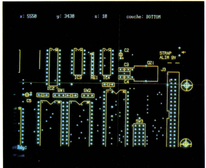
Plan de perçage + marque de sérigraphie.
