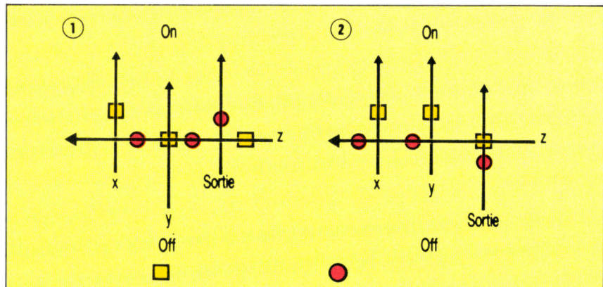
Figure A, ci-dessus : structure d'un bouton d'attente, structure d'un bouton de confirmation. Figure B, ci-dessous : (□ boutons d'attente, ● bouton de confirmation) représentation d'une porte NON-ET.
