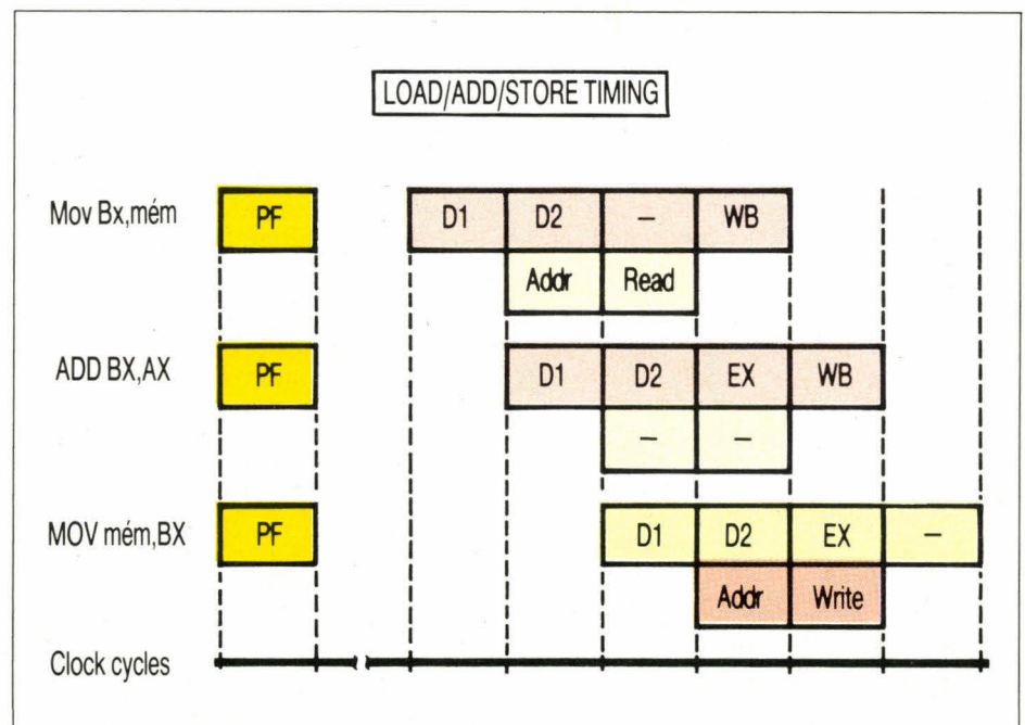
Fig. 2. - Etapes de pipeline pour une série de trois instructions à cycle unique. La première instruction est un simple chargement à partir de la mémoire et suppose la présence des données dans le cache ; les boîtes situées en dessous des étapes D 2 et EX montrent les actions de l'unité d'exécution (EU) et de la logique de cache à chaque cycle d'horloge. La seconde instruction effectue une addition de registre, en utilisant les données qui viennent d'être chargées et la troisième instruction est une instruction de stockage qui renvoie le résultat sur le même emplacement mémoire. Les trois instructions sont présélectionnées (prefetch) simultanément et chacune utilise un seul cycle d'horloge à chaque étape du pipeline.
