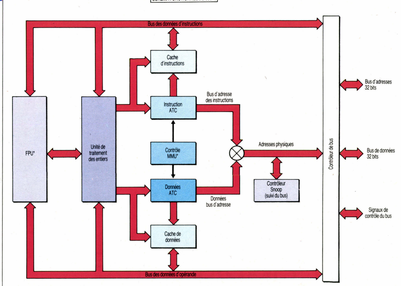
Fig. 5. - L'unité d'instructions du 68040 exécute le même jeu d'instructions que celle du 68030, avec peut-être quelques additions pour le support des nouvelles fonctionnalités matérielles. Cependant, la mise en œuvre est totalement nouvelle, avec une unité arithmétique et logique et un pipeline totalement reconçus pour diminuer le nombre moyen de cycles d'horloge par instruction. La taille de chacun des caches intégrés passe de 256 octets à 4 Ko. L'unité de traitement des calculs en virgule flottante (FPU) est intégrée à la puce.
