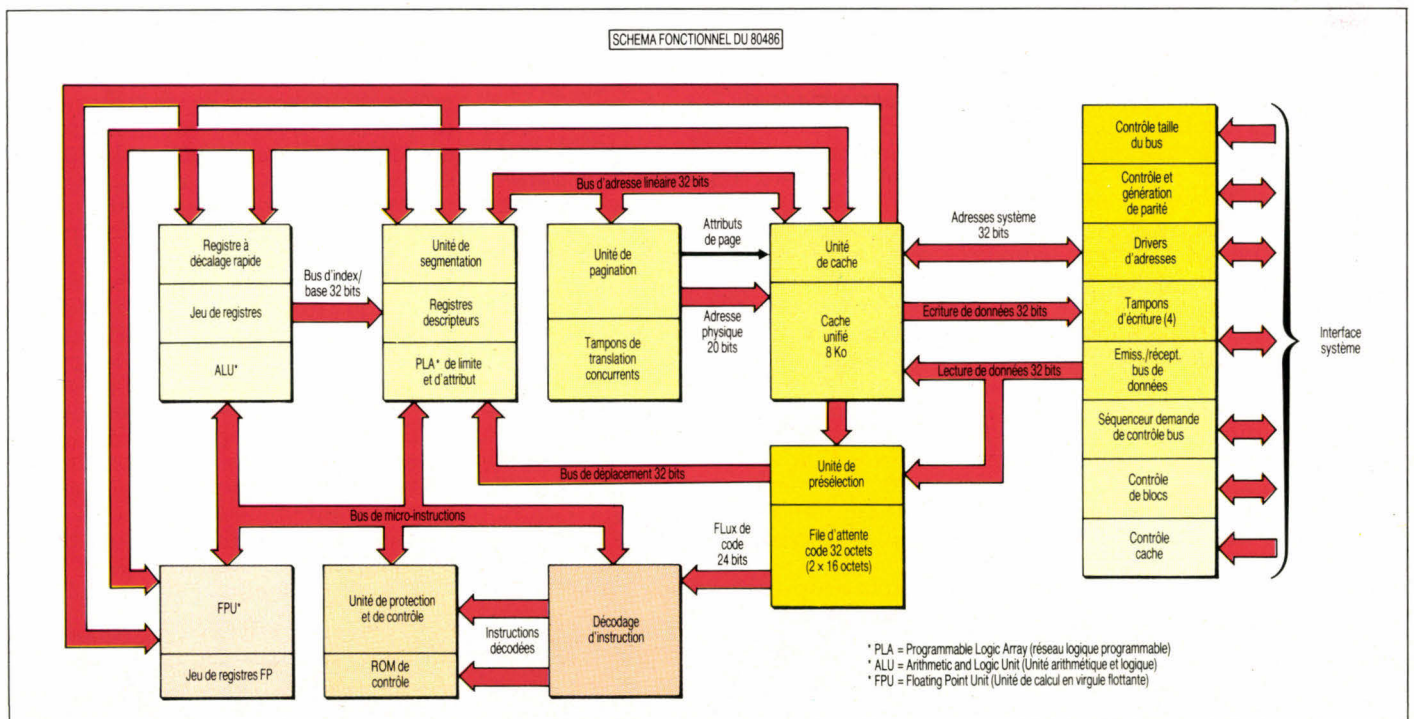
Fig. 1. - Le 486 utilise une technologie C.MOS ultrarapide (1 µ entre canaux) et contient 1,18 million de transistors. Ses performances, par comparaison avec le VAX 11/780, se situent entre 15 et 20 Mips VAX.
