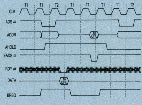
Fig. B. - La logique du système active d'abord AHOLD (address hold) puis le 80486 désactive ses sorties d'adresse sur le cycle d'horloge suivant. La logique du système dirige ensuite l'adresse sur les broches d'adresse du 80486 et active EADS# (external address). Si l'adresse fournie correspond aux références de cache, le 80486 invalide cette ligne de cache.
