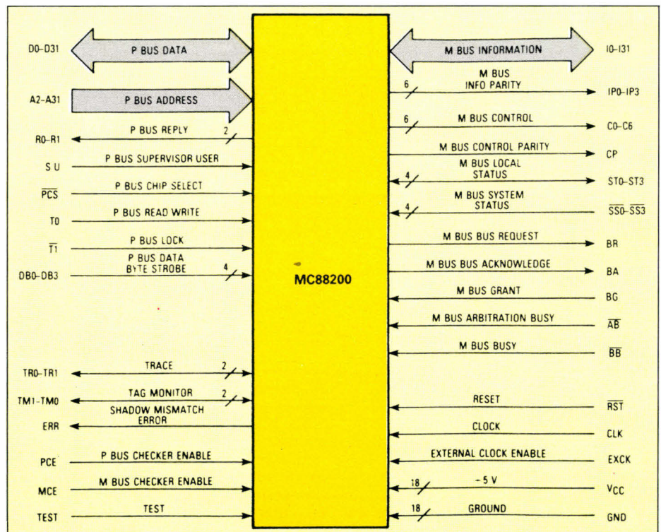
Schéma fonctionnel des signaux du MC 88200.
