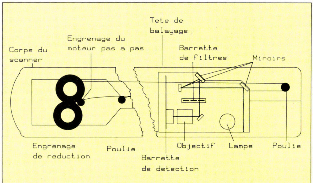
Fig. 1. - Pour produire une image couleurs, les poulies déplacent la tête de balayage du JX-100 au-dessus de l'original à trois reprises, de façon à échantillonner séparément les informations relatives aux couleurs rouge, vert et bleu.
