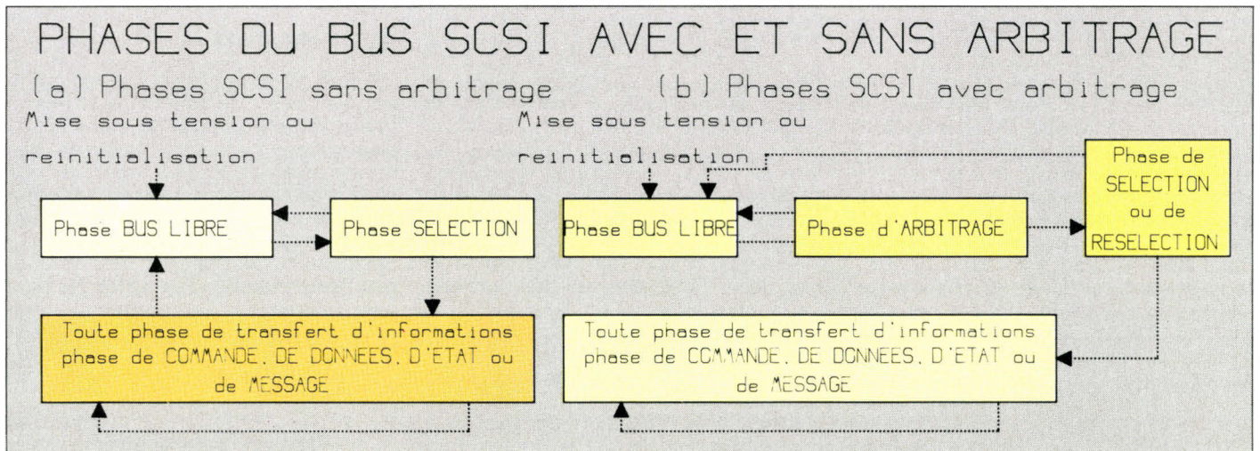
Fig. 3. - Le bus SCSI revient toujours en phase de BUS LIBRE. Un système peut être sans arbitrage (a) ou avec arbitrage (b) ; si l'arbitrage n'est pas mis en œuvre, il n'y a pas de phase d'ARBITRAGE ni de RESELECTION. Les systèmes sans arbitrage comprennent habituellement un seul système central et un seul contrôleur de périphériques ; l'ARBITRAGE et la RESELECTION sont alors inutiles car le système central a toujours le contrôle du bus, et les opérations de déconnexion/reconnexion ne sont pas nécessaires.
