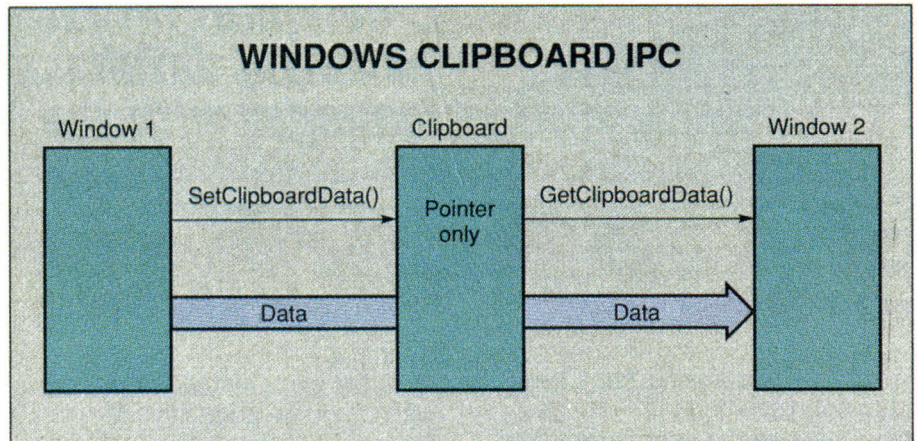
Fig. 2. - IPC du presse-papiers de Windows. La fenêtre 1 place un pointeur vers les données situées dans le presse-papiers où la fenêtre 2 peut les prendre et les déplacer en une seule opération.
