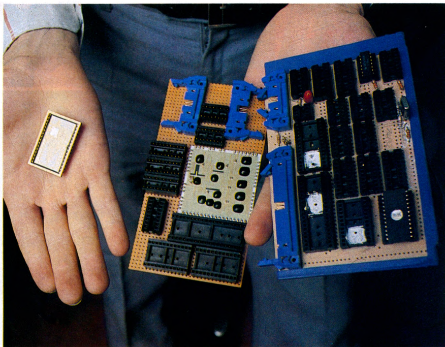
Les trois étapes de la conception du circuit intégré du Cyborg. A droite, la carte prototype : les circuits intégrés sont dans plusieurs boîtiers. Au centre, la carte hybride : plusieurs circuits intégrés sont réunis dans un seul boîtier. A gauche, l'étape finale : les puces du circuit hybride sont fondus en un seul circuit intégré.
