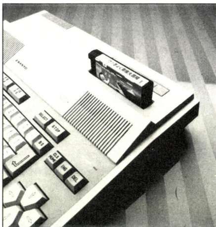
Les ordinateurs familiaux MSX privilégient les logiciels sur cartouches par rapport à ceux sur cassettes. Le Sanyo PHC 28 possède deux connecteurs de cartouches.
