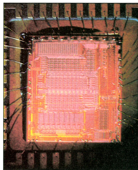
Le cœur d'un Apple II (Microprocesseur 6502) grossi 3 fois.
