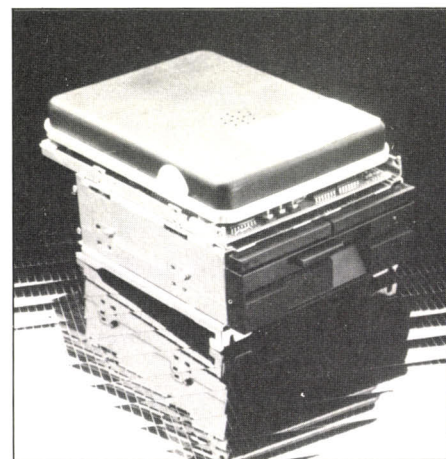
Le disque dur miniaturisé au sommet du lecteur de disquettes.
