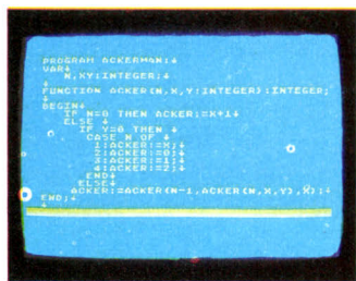
Le PASCAL: un langage d'analyse informatique.
