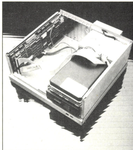
A droite, le lecteur de disquettes mi-hauteur et, au-dessus, le disque dur.
