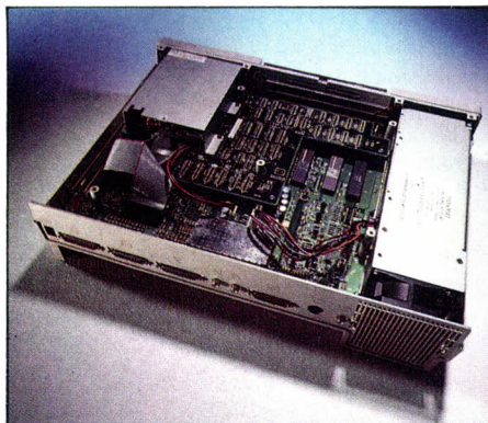
L'intérieur de l'Amiga : sur la carte de base, on distingue les trois processeurs spéciaux qui gèrent les périphériques et le graphisme.
