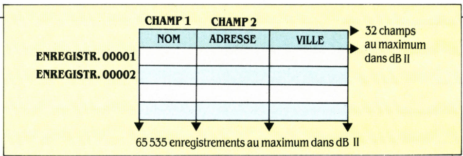
Schéma 1. Un fichier dBase II : un tableau à deux dimensions.
