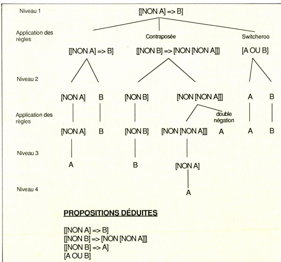
Exemple de déduction à partir d'une expression composée. À chaque niveau le programme applique les règles possibles puis décompose chaque terme obtenu pour passer au niveau suivant.
