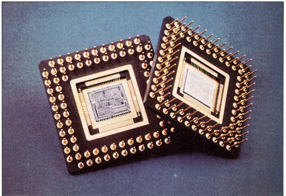
Le NS 32332 a un boîtier « en tapis de fakir », rendu indispensable par le nombre de connecteurs.
