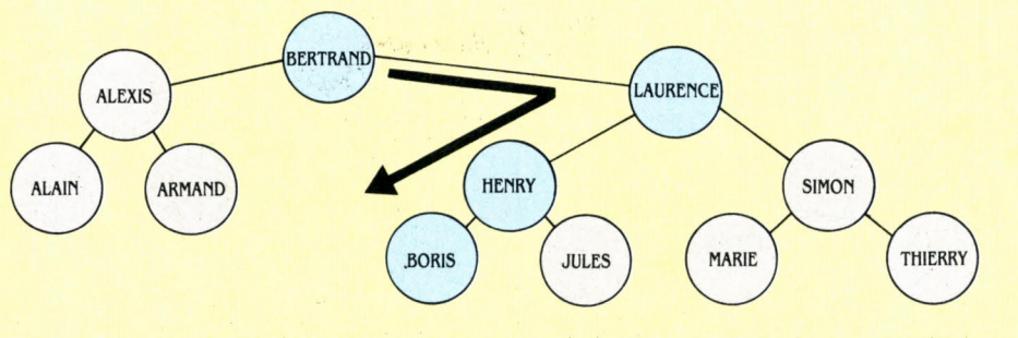
Schéma 3. L'indexation en arbre suppose que si la donnée recherchée est plus grande que la valeur du nœud, la recherche est poursuivie vers la branche de droite et si la valeur est plus petite, vers la branche de gauche. Ici, pour rechercher le nom « Boris », tout le cheminement indiqué en couleur doit être parcouru.
