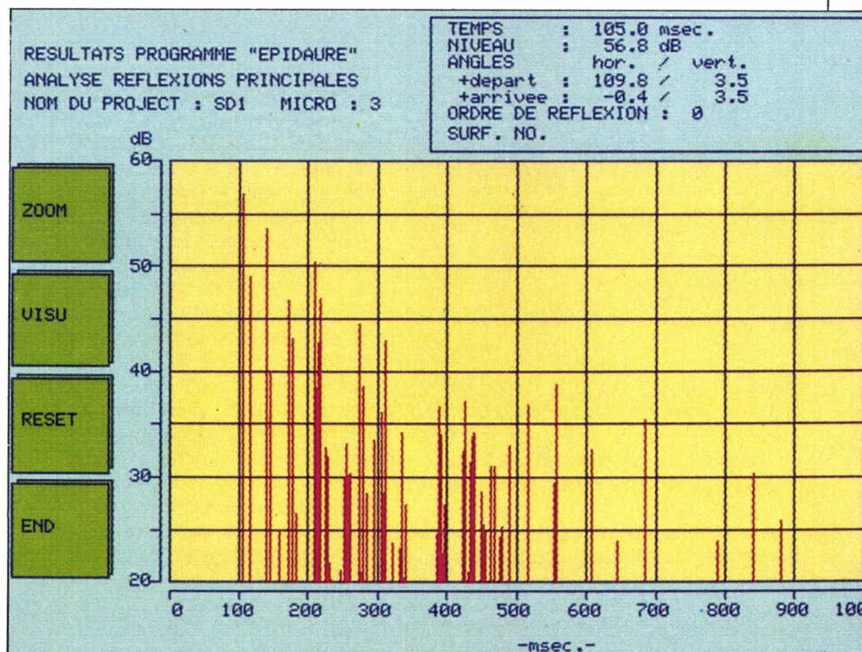
Une autre représentation (ci-dessus) montre, dans les instants qui suivent son émission, à quelle puissance le son se réfléchit sur les parois.
