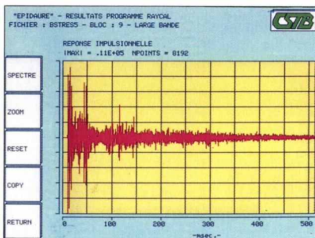
L'analyse de la réponse impulsionnelle (graphique 4 ci-dessus) permet de visualiser la décroissance d'un son dans le temps.
